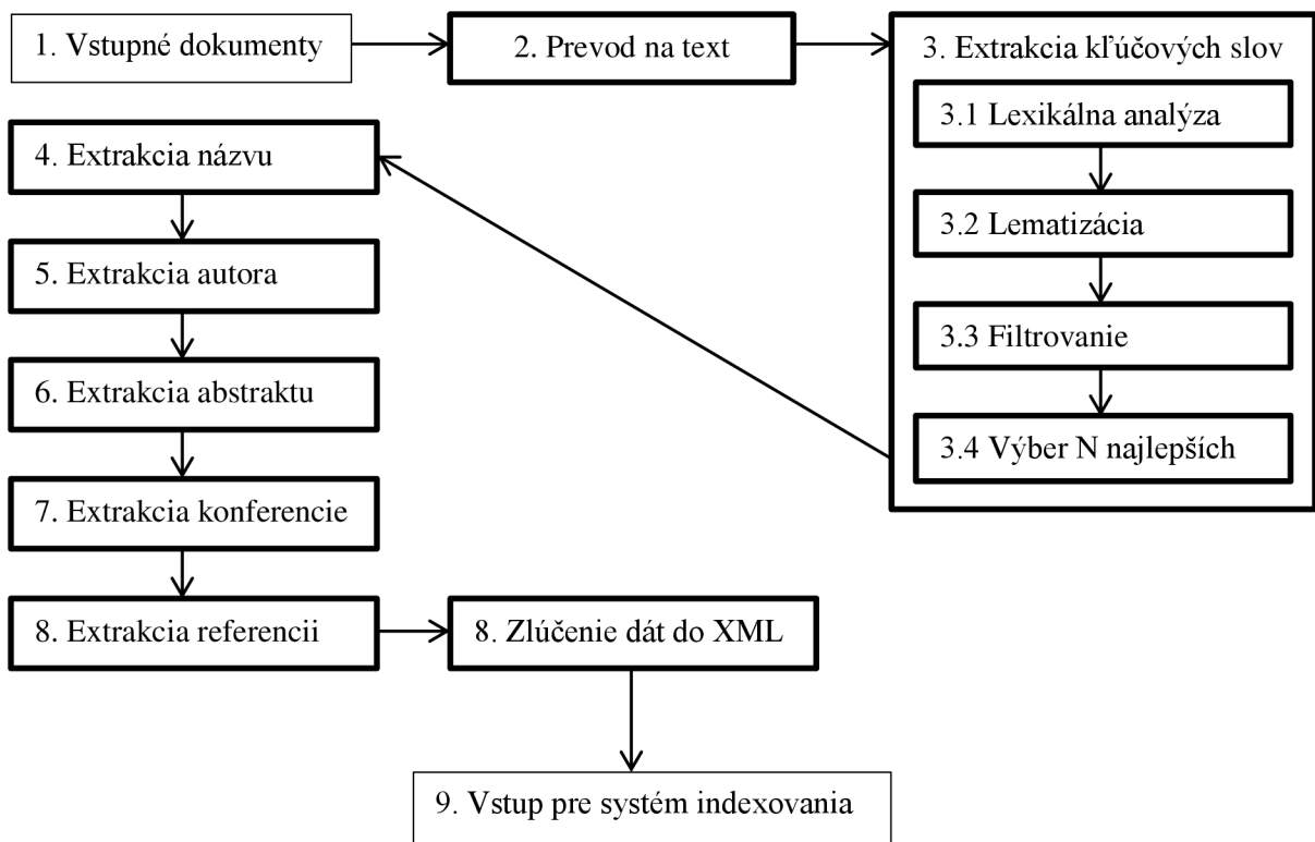
Obrázok 4.1: Návrh systému pre pedspracovanie dokumentov
