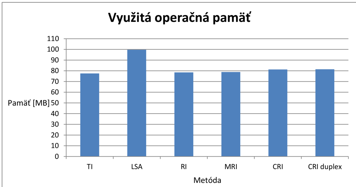
Obrázok 6.3: Graf využitej operačnej pamäte
