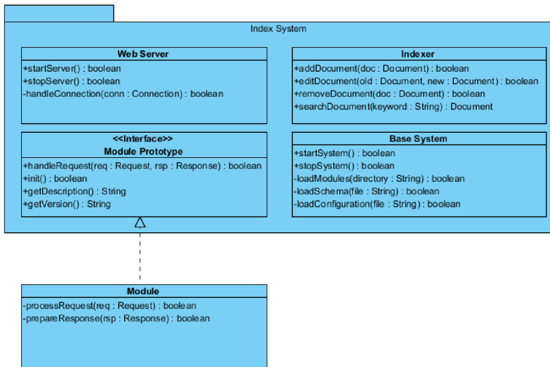
Obrázok 4.2: Vizualizácia návrhu systému pre indexovanie
