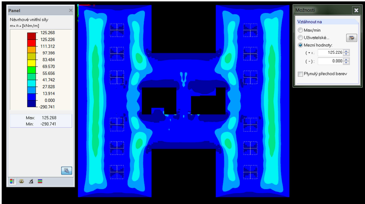
Obr.15 Dimenzační momenty m_x, D+
