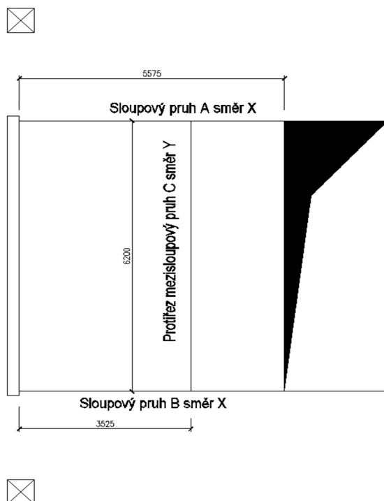
Obr.23 Umístění řezů
