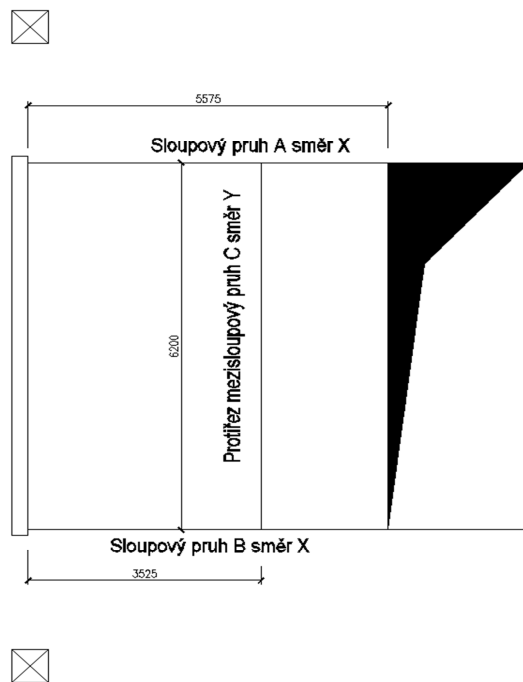
Obr.12 Umístění řezů
