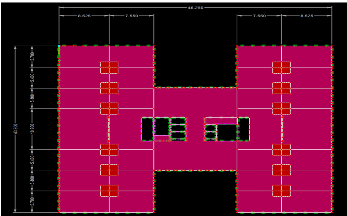
Obr.14 Základní rozměry
