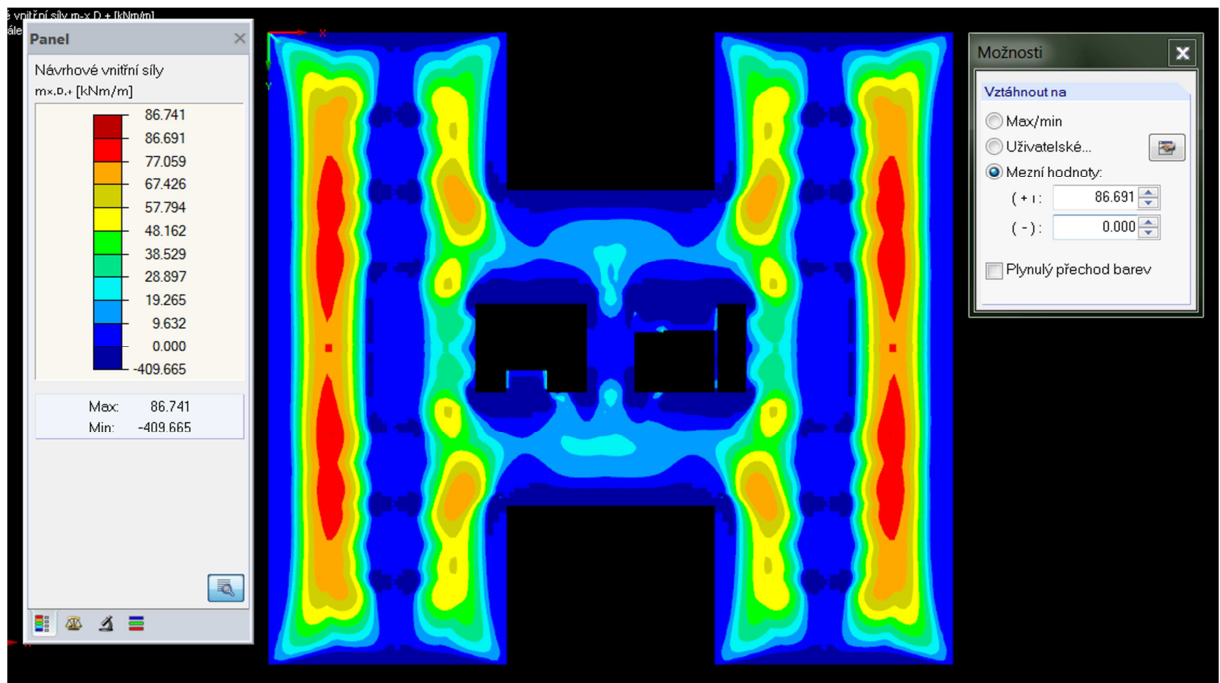
Obr.26 Dimenzační momenty m_{x,D+}
