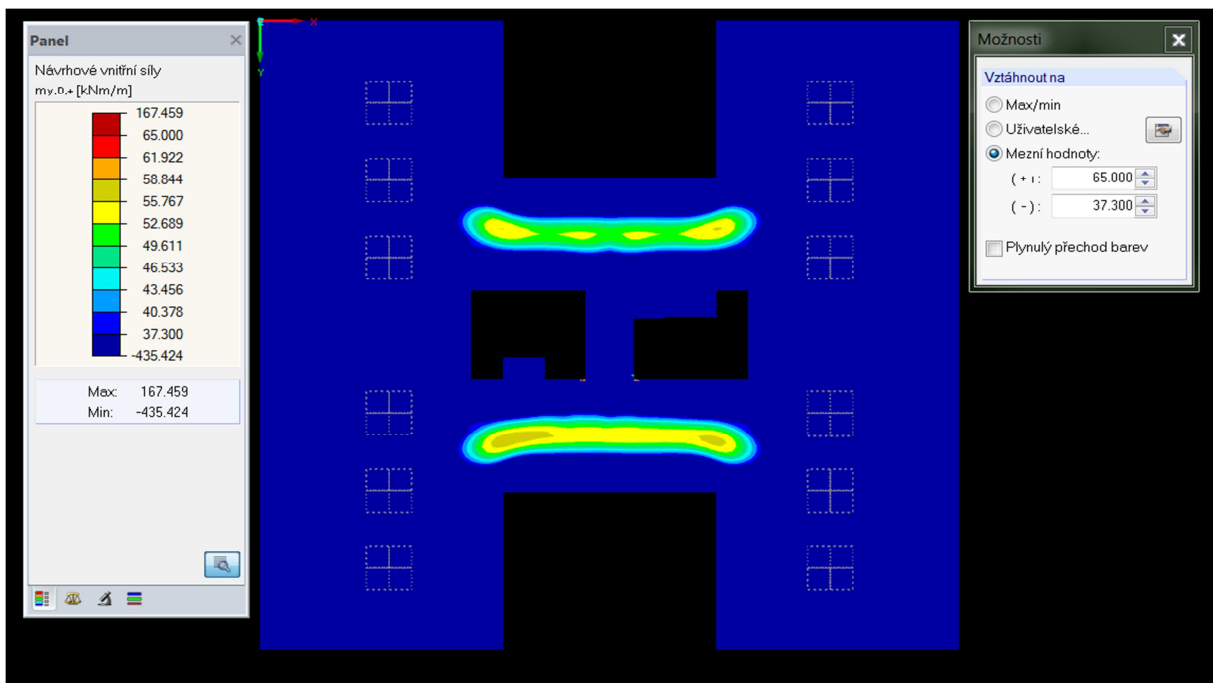
Obr.18 Výsledky vnitřních sil po uvažování základní sítě ve směru y
