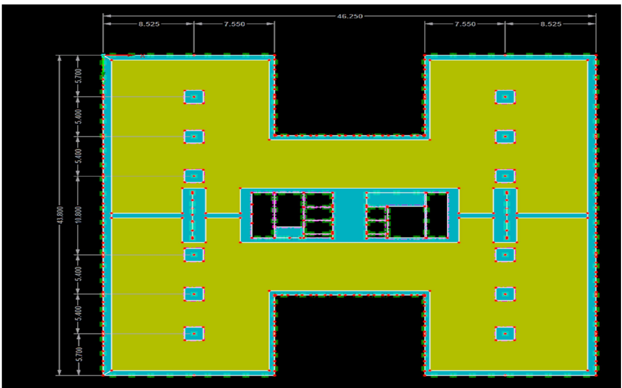
Obr.25 Základní rozměry
