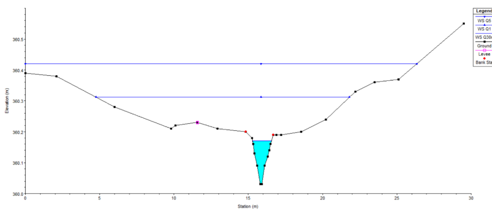
Obr. 32 PF 300, úsek, kde potok nevybřeží při Q_{30} (HEC-RAS)
