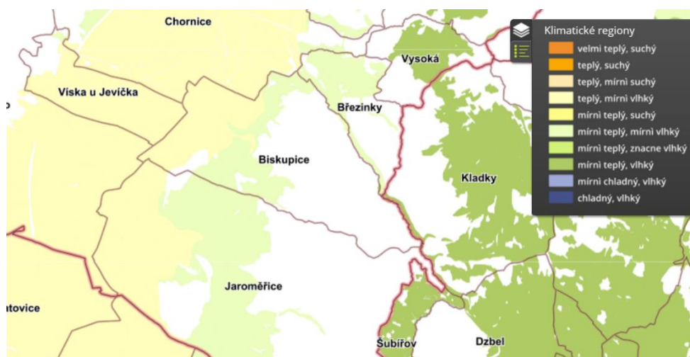
Obr. 20 Mapa klimatických regionů [24]
