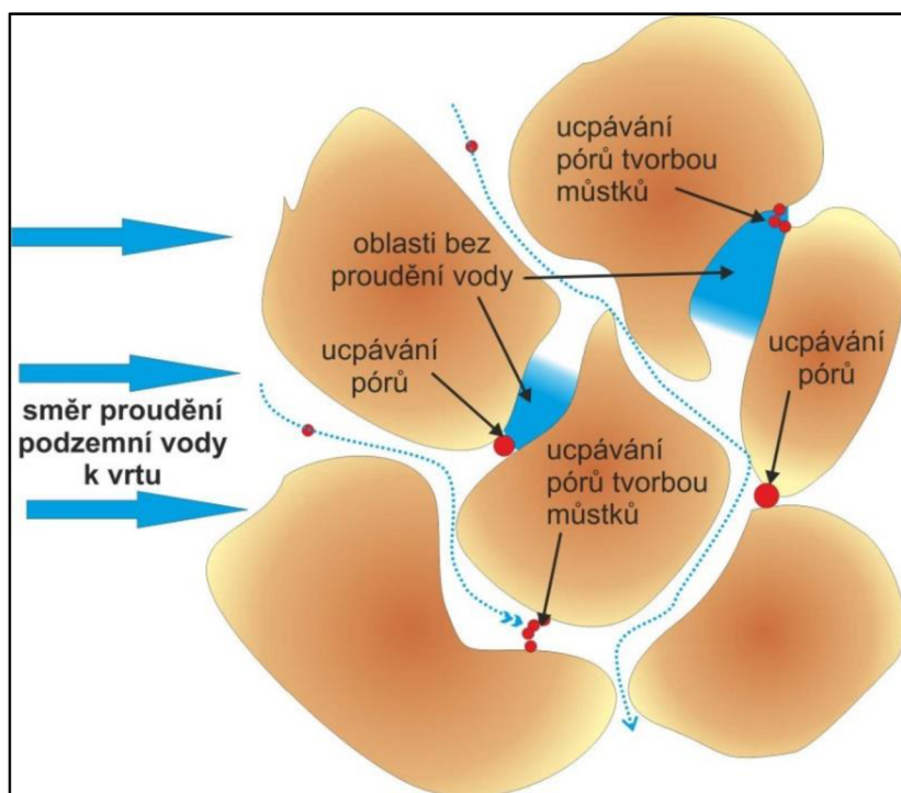
Obrázek 6. Schematizovaný mechanismus kolmatace obsypu vrtu (archiv autora)
