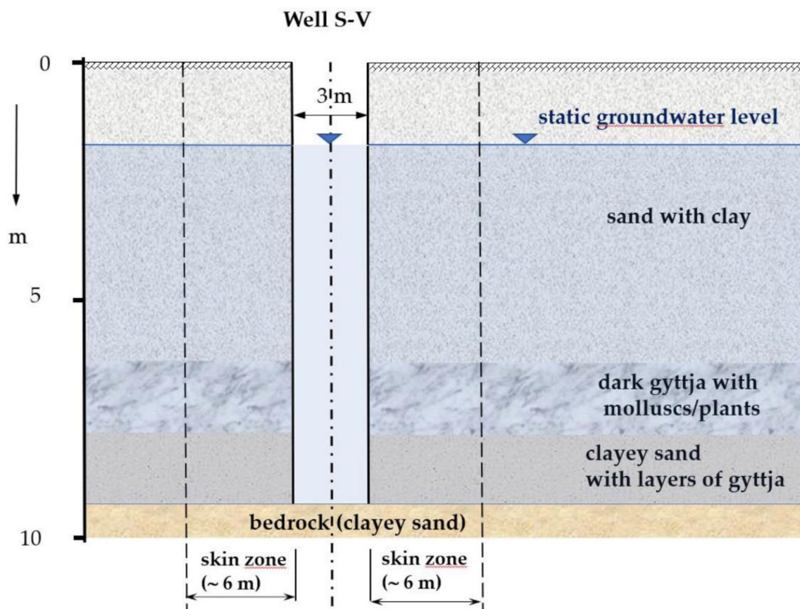
Figure 10. Cross-section of the S-V well with geology (Hošek, Pokorný, Prach, Šída, & Křížek, 2018).
