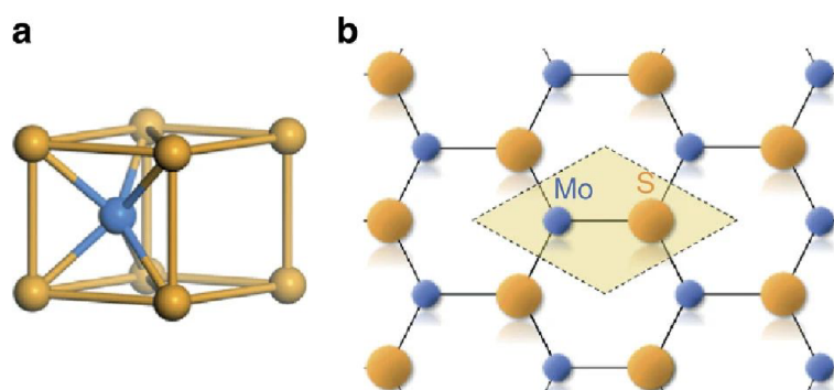
Obrázek 1.1: Krystalová struktura MoS 2 a) pohled na koordinační prostředí molybdenu. b) Monovrstva MoS 2 z pohledu shora s vyznačenou primitivní buňkou. Atomy molybdenu jsou vyznačeny modře, atomy síry žlutě. Převzato z [22].
