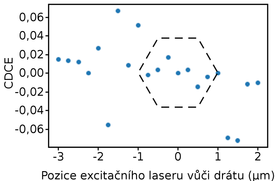
Obrázek 6.4: Graf CDCE naměřené za pokojové teploty. Černý přerušovaný šestiúhelník znázorňuje polohu ZnO vlnovodu.
