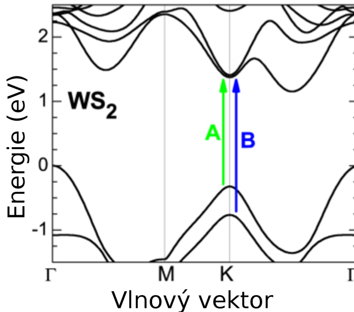
Obrázek 2.1: Simulovaný průběh pásové struktury WS 2 . Pomocí zelené a modré šipky jsou zde znázorněny optické přechody A a B (popsané v části 1.2) mezi rozštěpenými hladinami vodivostního a valenčního pásu. Toto rozštěpení je důsledkem SOI elektronů. Převzato a upraveno z [49].
