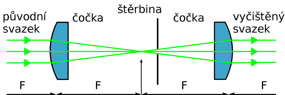
Obrázek 5.2: Schéma prostorového filtračního systému. V blízkosti společného ohniskového bodu dvou čoček (označeného šipkou) je umístěna úzká štěrbina, která filtruje procházející svazek (zelené čáry). Velké písmeno F představuje ohniskovou vzdálenost čoček. Převzato a upraveno z [69].
