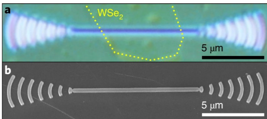
Obrázek 3.2: Snímky pořízené pomocí a) optického mikroskopu a b) rastrovacího elektronového mikroskopu zobrazují nanofotonické zařízení, které je určeno ke směrovému šíření světla. Součástí struktury zařízení jsou mřížkové antény pro lepší navazování/vyvazování světla z konců vlnovodu. V prvním obrázku je pomocí žluté čáry vyznačena oblast, kde se nachází monovrstva \text{WSe}_2 . Převzato a upraveno z [56]
