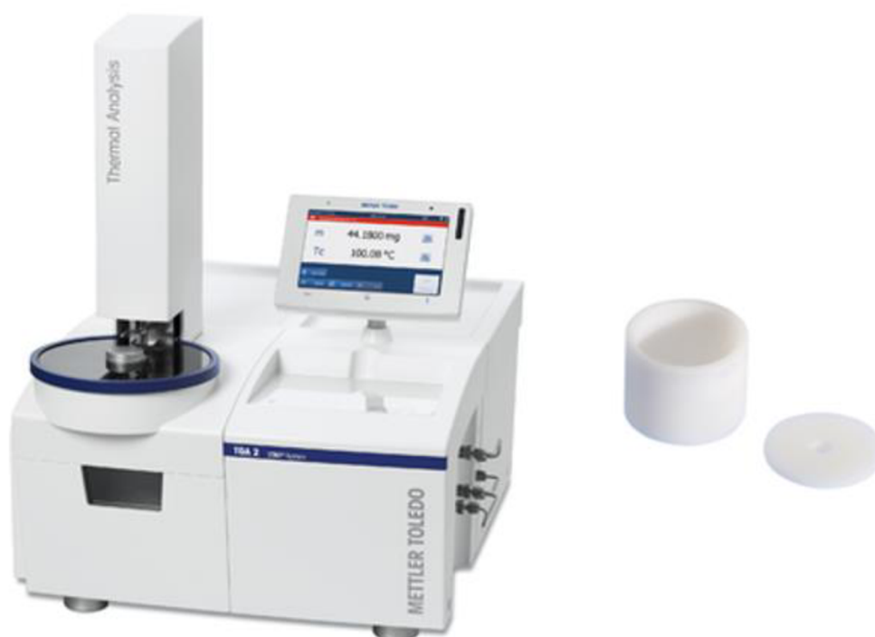
Obr. 3.19 - Přístroj Mettler Toledo TGA 2 (vlevo) a kelímky na vzorky (vpravo) [56]
