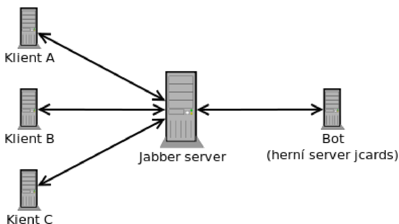
obr 4.1: komunikace jcards
