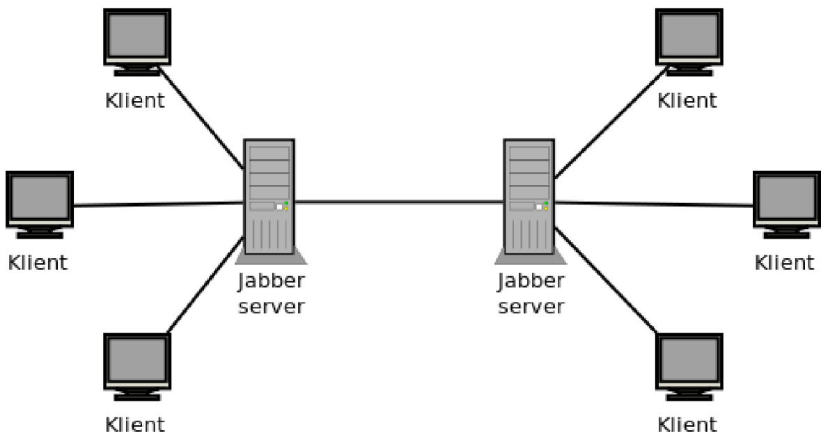
obr 2.1: architektura jabberu
