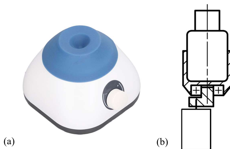
Obr. 2-6 (a) Vortexová míchačka [8]; (b) Znáznornění funkce
