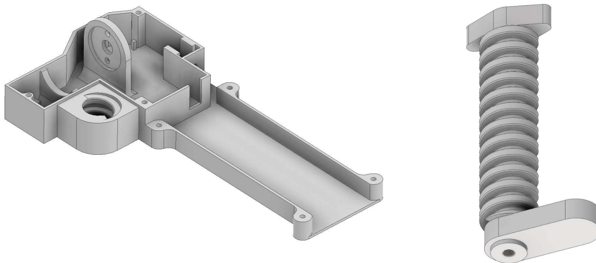
Obr. 5-17 (a) Tělo míchačky doplněné o závit; (b) Svěrka
