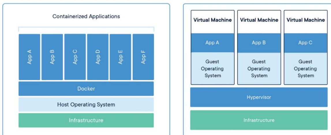
Obrázek 9: Diagram srovnávající Docker kontejnery a virtualizaci. [26]
