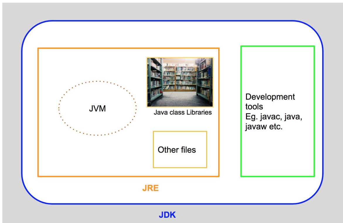
Obrázek 6: JDK Diagram [13]
