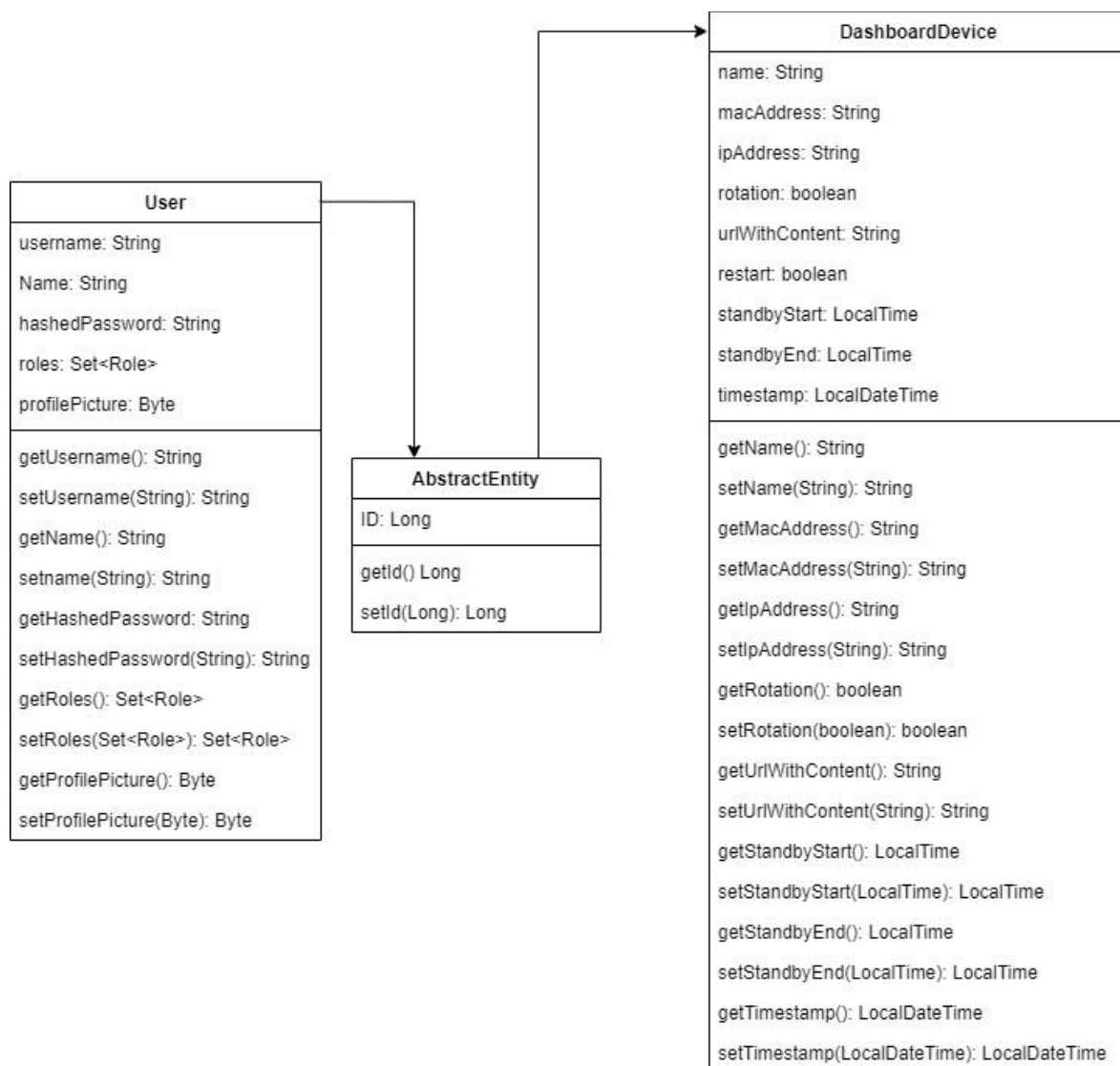
Obrázek 15: Diagram tříd
