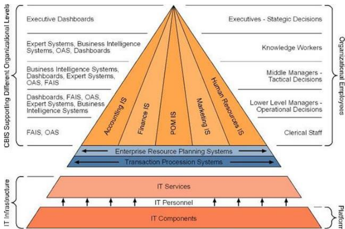
Obrázek 1: Architektura IS [4]
