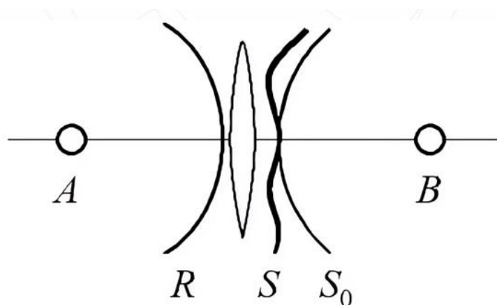
Obrázek 13: Porucha vlnoplochy (upraveno) [12]
