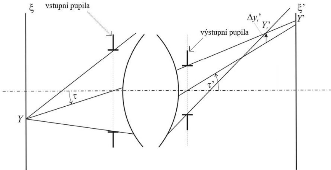
Obrázek 7: Tangenciální koma (upraveno) [2]
