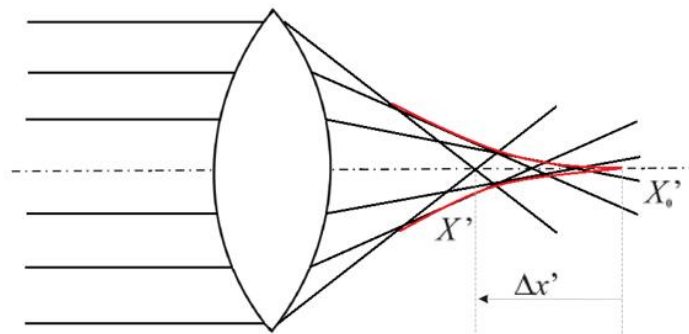
Obrázek 4: Kaustika (upraveno) [4]
