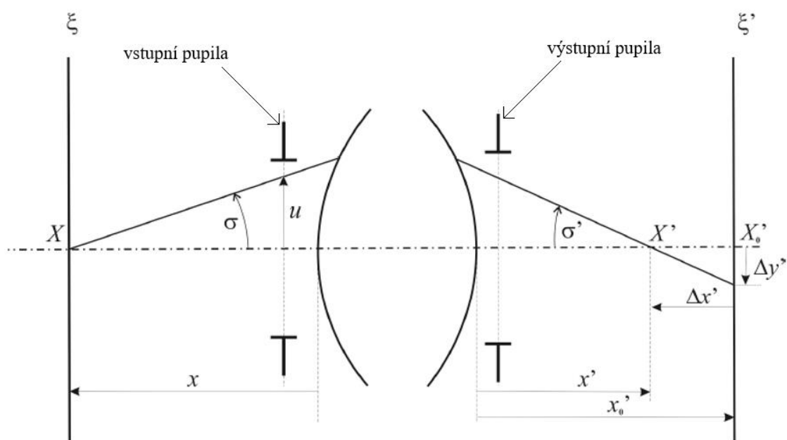
Obrázek 3: Otvorová vada (upraveno) [2]
