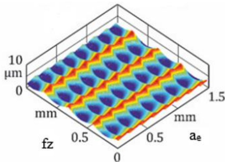
Obrázek 45 Rozdílná drsnost povrchu v důsledku rozdílné hodnoty kroku a posuvu [34].
