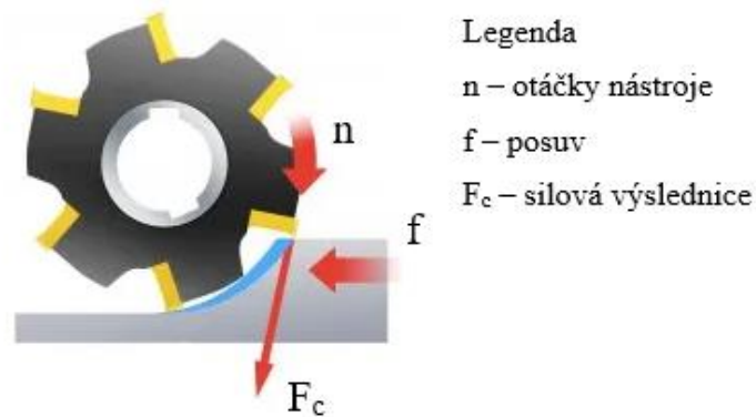
Obrázek 9 Kinematika při sousledném frézování upraveno dle [26].
