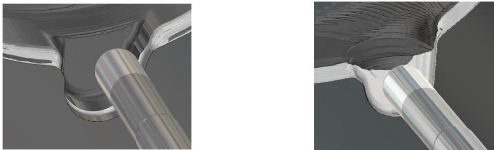
Obrázek 31 Porovnání množství odebíraného materiálu pro dokončení hrubování kruhového vybrání.
