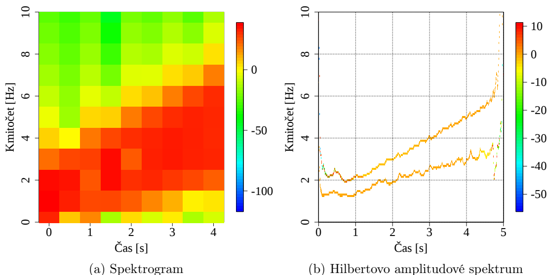
Obr. 1.14: Srovnání spektrogramu s Hilbertovým amplitudovým spektrem
