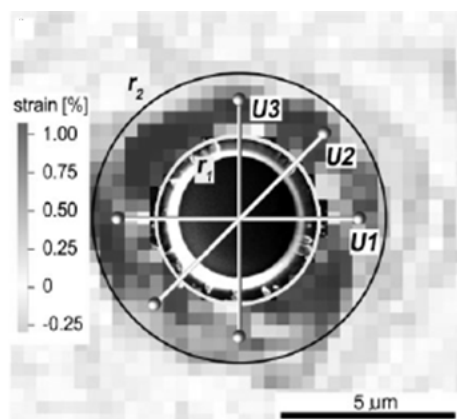
Obr. 3.1: Body pro určování posuvů, převzato z [19]
