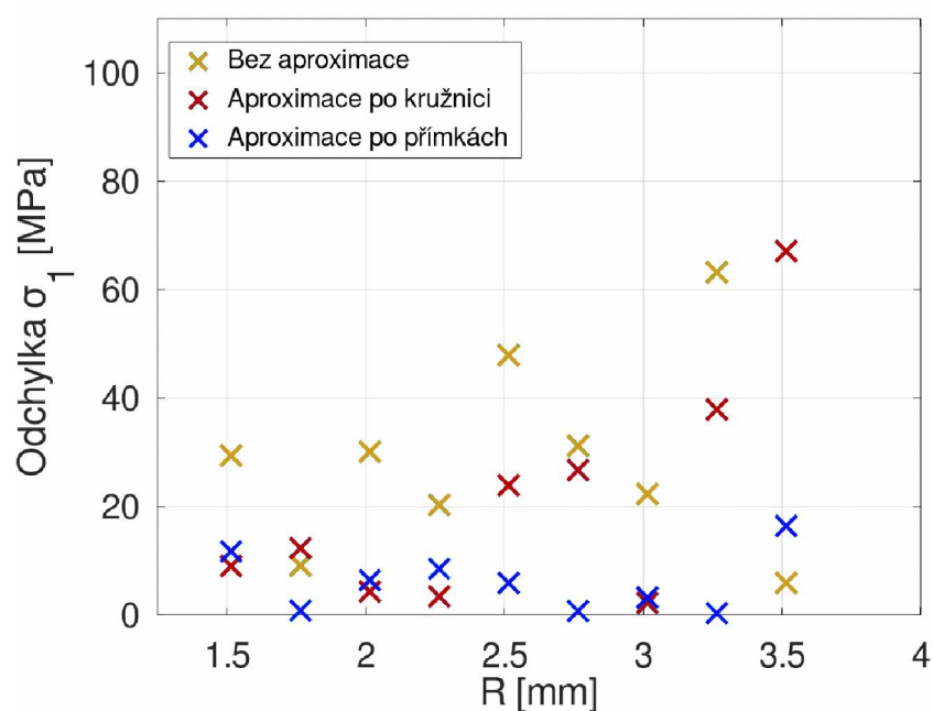
Obr. 7.38: Vykreslení absolutních odchylek zbytkového napětí \sigma_1 v závislosti na poloměru kružnice R
