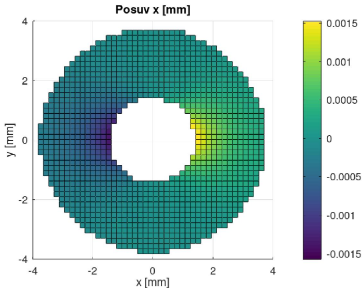
Obr. 7.21: Posuvy ve směru osy x pro hloubku otvoru 1\text{ mm} , jedná se o případ D
