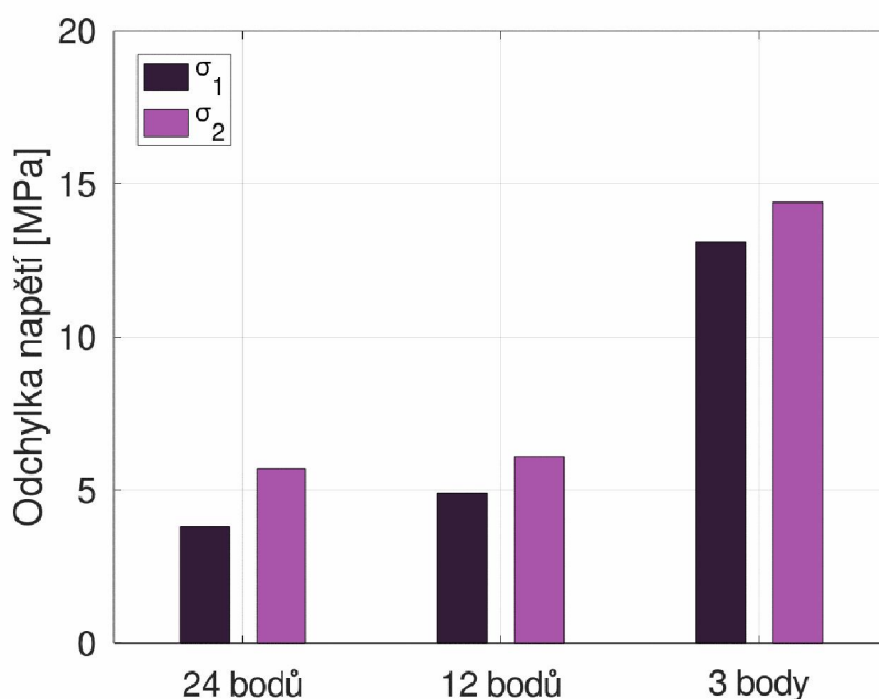
Obr. 7.16: Porovnání průměrných odchylek hlavních napětí pro různé metody výpočtu pro hloubku otvoru 0,5 mm
