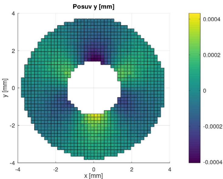
Obr. 7.22: Posuvy ve směru osy y pro hloubku otvoru 1\text{ mm} , jedná se o případ D
