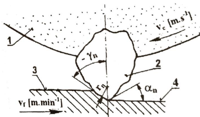
Obr. 15 Model záběru brousícího zrna [29].
