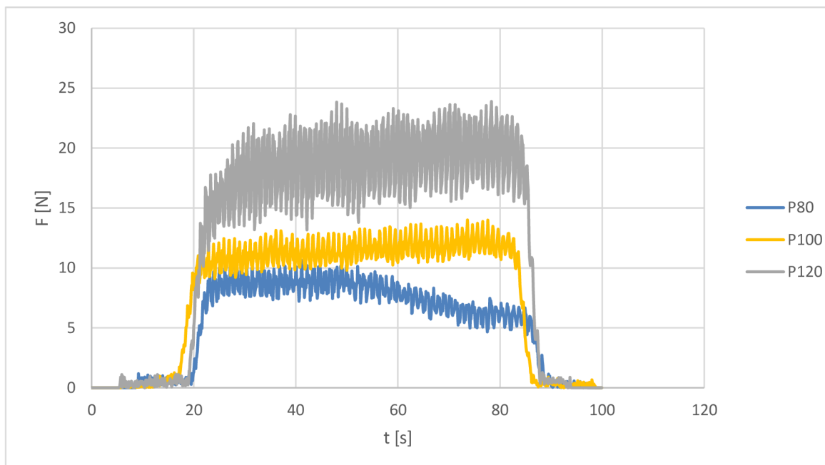
Obr. 37 Graf celkové síly při obrábění při hloubce broušení a_p=0,1 mm.
