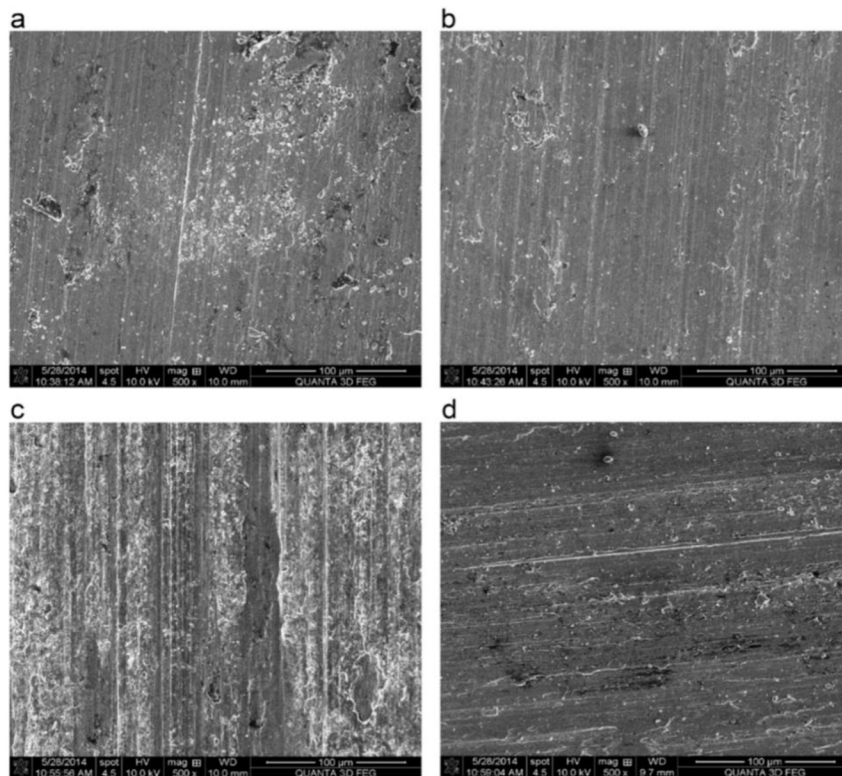
Obr. 12 Mikroskopické snímky povrchu Ti-6Al-4V po broušení podle druhu mazání a) bez mazání, b) MWF mazání, c) MQL mazání s nanočásticemi z \text{Al}_2\text{O}_3 , d) MQL mazání s nanočásticemi z \text{CuO} [25].
