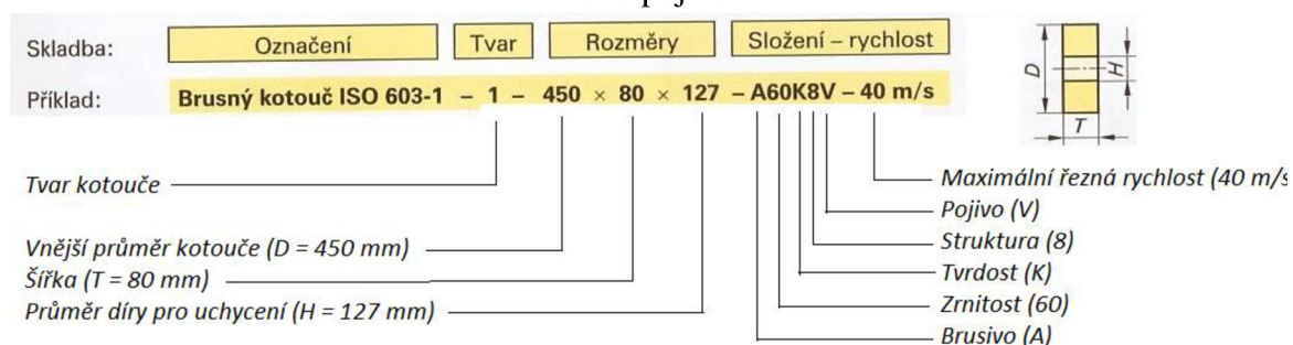
Obr. 21 Značení brousících kotoučů [39].
