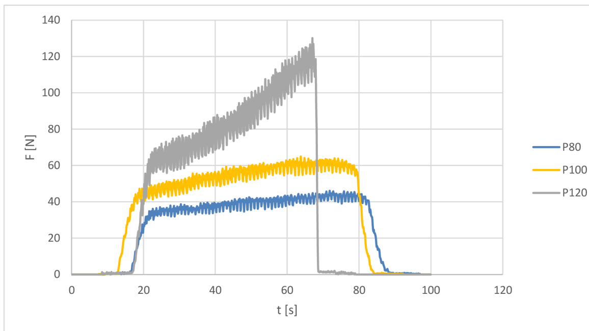
Obr. 39 Graf celkové síly při obrábění při hloubce broušení a_p=0,3 mm.
