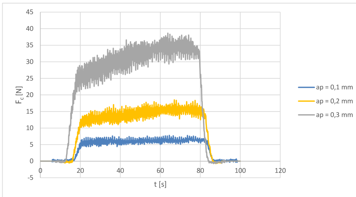
Obr. 29 Graf řezné síly při zmitosti pásu P100.
