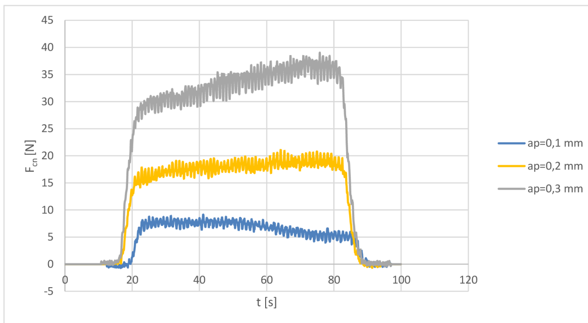
Obr. 34 Graf kolmé řezné síly při zmitosti pásu P80.
