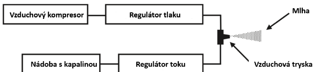
Obr. 10 Schématický diagram stroje pro MQL [26].
