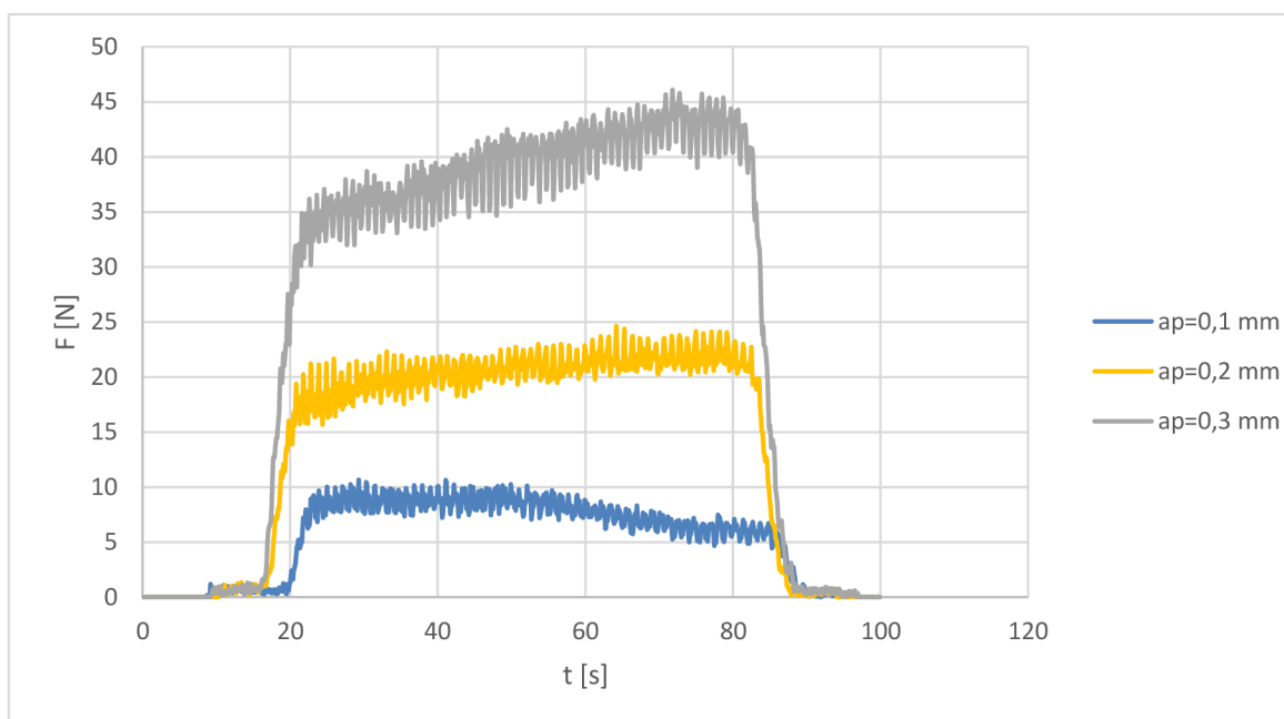
Obr. 40 Graf celkové síly při obrábění při zmitosti pásu P80.
