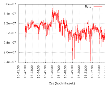
Obrázek 6.10: Počet bytů.
