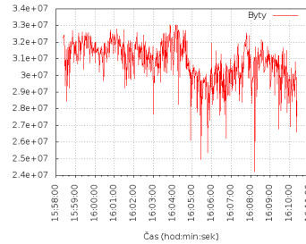
Obrázek 6.6: Počet bytů.
