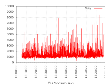
Obrázek 6.23: Počet toků.
