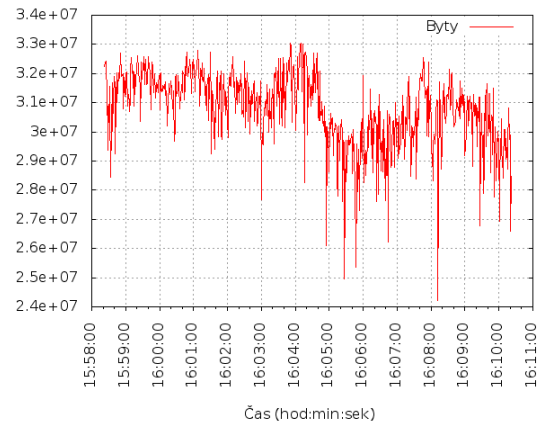
Obrázek C.5: Počet bytů.
