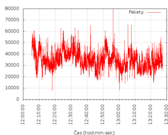
Obrázek 6.21: Počet paketů.
