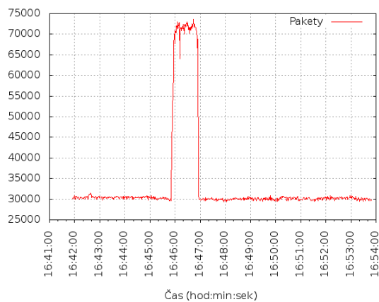
Obrázek C.7: Počet paketů.
