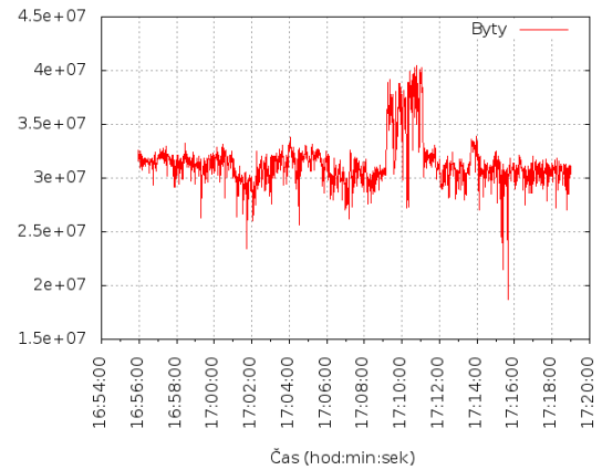
Obrázek C.11: Počet bytů.
