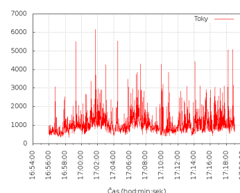
Obrázek 6.15: Počet toků.
