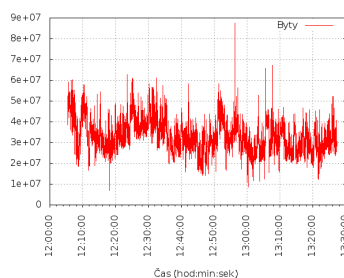
Obrázek 6.22: Počet bytů.
