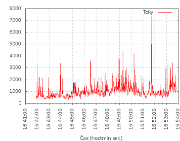
Obrázek 6.11: Počet toků.
