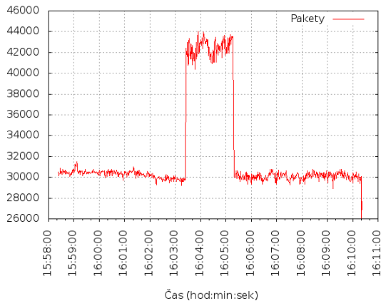
Obrázek C.4: Počet paketů.
