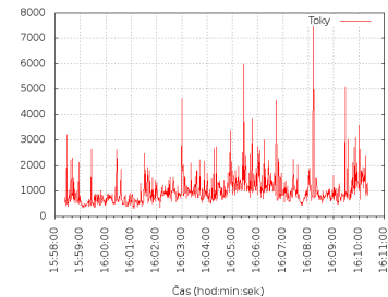
Obrázek 6.7: Počet toků.
