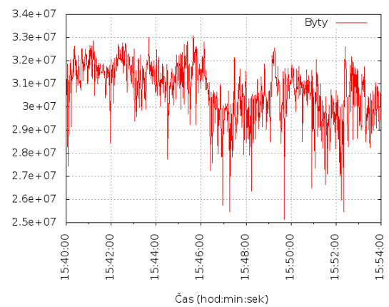
Obrázek C.2: Počet bytů.
