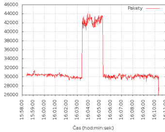
Obrázek 6.5: Počet paketů.
