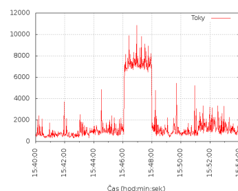
Obrázek 6.3: Počet toků.
