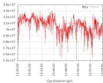
Obrázek 6.2: Počet bytů.
