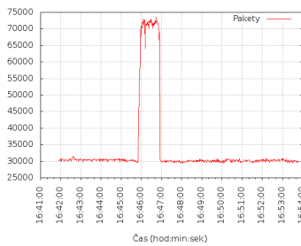
Obrázek 6.9: Počet paketů.
