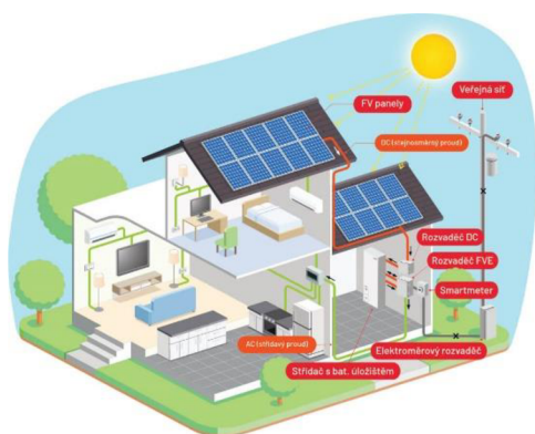
Obr. 1 – Fotovoltaická elektrárna – schéma
