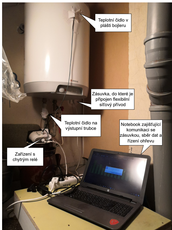
Obrázek 5.4: Instalace zařízení pro sběr dat v domácnosti s 80 litrovým bojlerem. Na snímku se nachází bojler, na který jsou připojena teplotní čidla, zařízení s chytrým relé a zásuvkou pro přívod elektrické energie bojleru. Dále pak notebook, na kterém se nachází služba Docker s kontejnery, zajišťujícími chod chytrého ohřevu jako je databáze nebo skripty pro sběr dat a řízení ohřívání.
