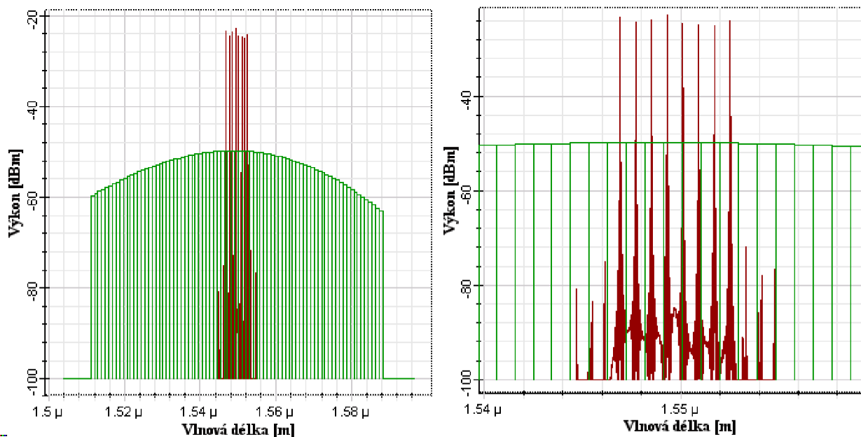
Obr. č. 17 Spektrum signálu a šumu předzesilovače SOA
