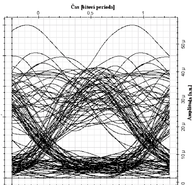
Obr. č. 18 Diagram oka ve scénáři s předzesilovačem SOA
