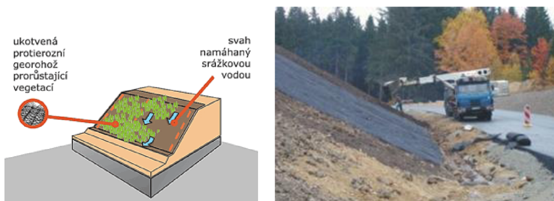
Obrázek 6: Aplikace georohože
