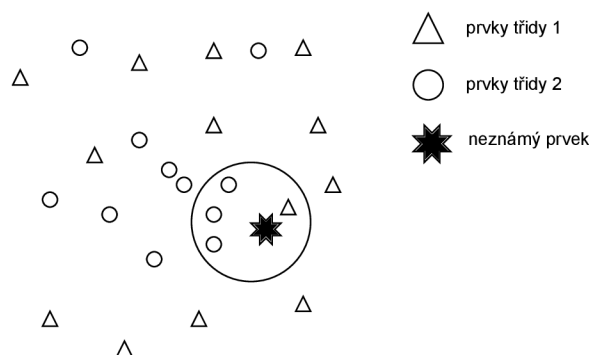
Obr. 3.6: Popis principu Algoritmu k-nejblížších sousedů
