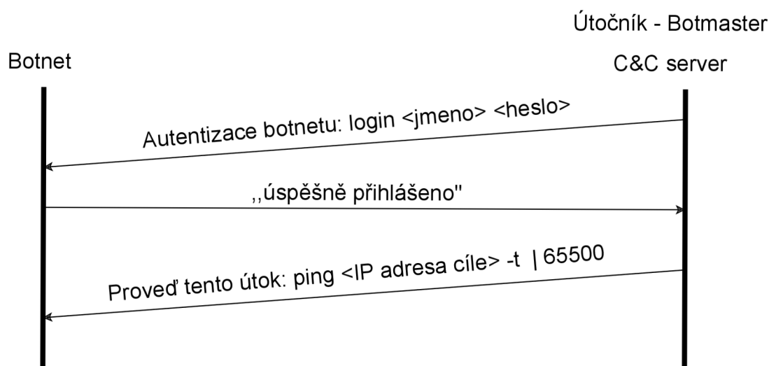
Obr. 1.2: Princip ovládnutí botnetu: útok Ping of death
