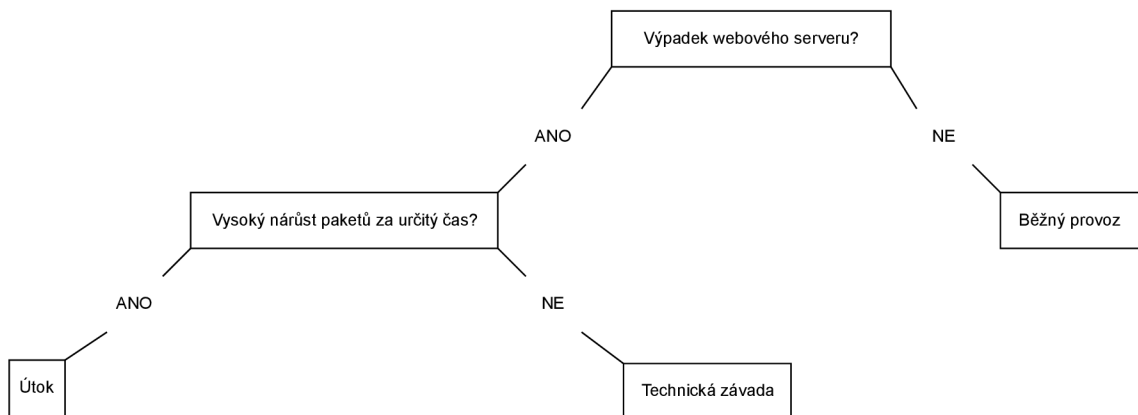
Obr. 3.5: Příklad analýzy provozu dle rozhodovacího stromu
