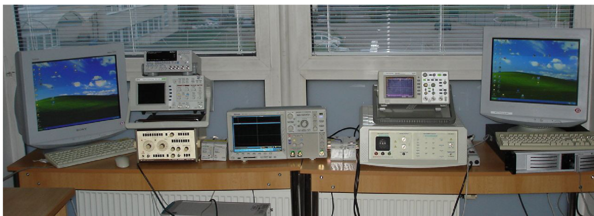
obrázek 7.1: Měřicí pracoviště.
