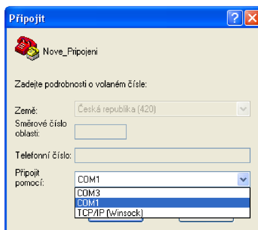
obrázek 8.3: Program Hyperterminál.
