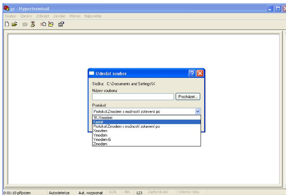
obrázek 8.6: Program Hyperterminál.
