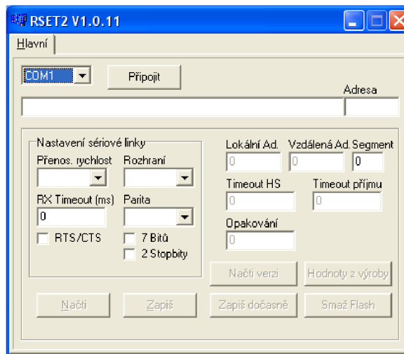
obrázek 8.1: Program RSET.
