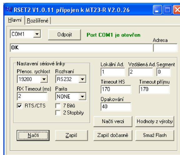
obrázek 8.2: Program RSET.
