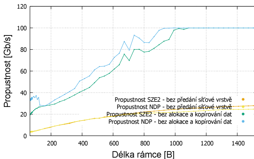
Obrázek 5.5: Srovnání dosažené propustnosti nad jediným RX DMA kanálem mezi modifikovanými ovladači pro SZE2 a NDP rozhraní. Modifikace odstraňuje alokaci paměti a kopírování dat při každém rámci, a díky tomu dosahuje téměř referenčních výsledků. Graf také obsahuje variantu ovladače bez předání rámce síťové vrstvě z předchozího grafu 5.4 pro porovnání.
