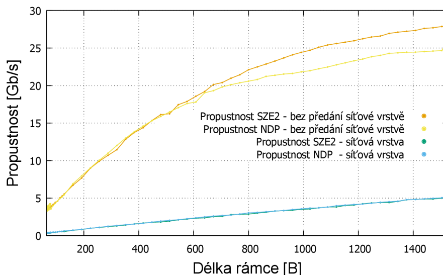
Obrázek 5.4: Srovnání dosažené propustnosti nad jediným RX DMA kanálem mezi ovladači pro SZE2 a NDP rozhraní. Graf zároveň zachycuje vliv zpracování rámce síťovou vrstvou na celkovou propustnost.
