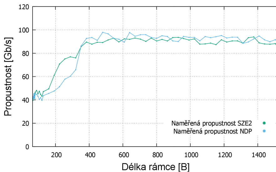
Obrázek 5.6: Referenční měření zachycující maximální možnou propustnost nad jediným TX DMA kanálem při použití nástrojů sze2fastwrite pro SZE2 a ndp-tool pro NDP rozhraní.
