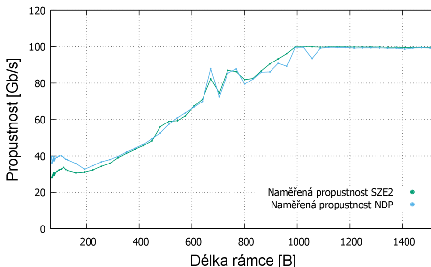
Obrázek 5.3: Referenční měření zachycující maximální možnou propustnost nad jediným RX DMA kanálem při použití nástrojů sze2multiread pro SZE2 a ndp-tool pro NDP rozhraní.
