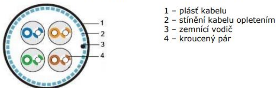
Obrázek 9: STP kabel
