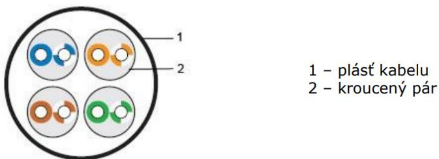
Obrázek 10: UTP kabel
