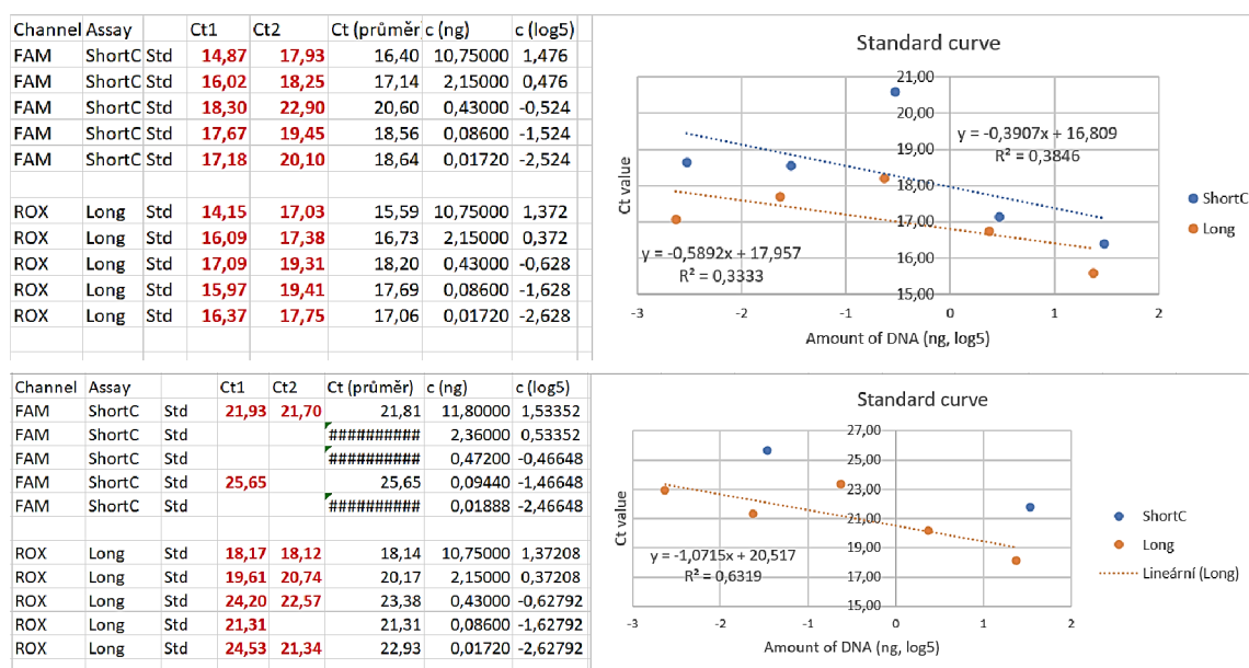
Obrázek 6 Ukázka standardů u experimentů č. 11 (výše) a 12 (níže) s podmínkami touchdown 70 °C–60 °C. Ve sloupcích Ct1 a Ct2 (duplikáty) je možné pozorovat ať už nesmyslné, či chybějící hodnoty pro standardy.
