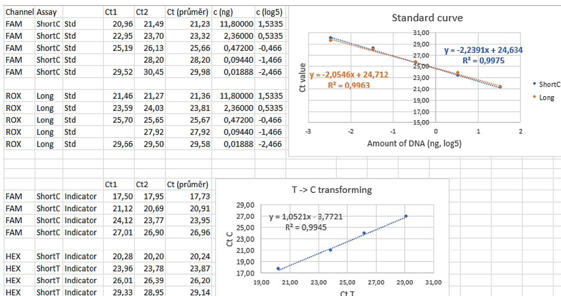
Obrázek 9 Ukázka standardů (výše) a C- T- indikátorů (níže) u experimentu pro evaluaci konverze vzorků po NEBNext a bisulfitové konverzi. Standardy i indikátory byly měřeny v duplikátech (Ct1 a Ct2). Ct hodnoty u standardů i indikátorů jsou v pořádku.
