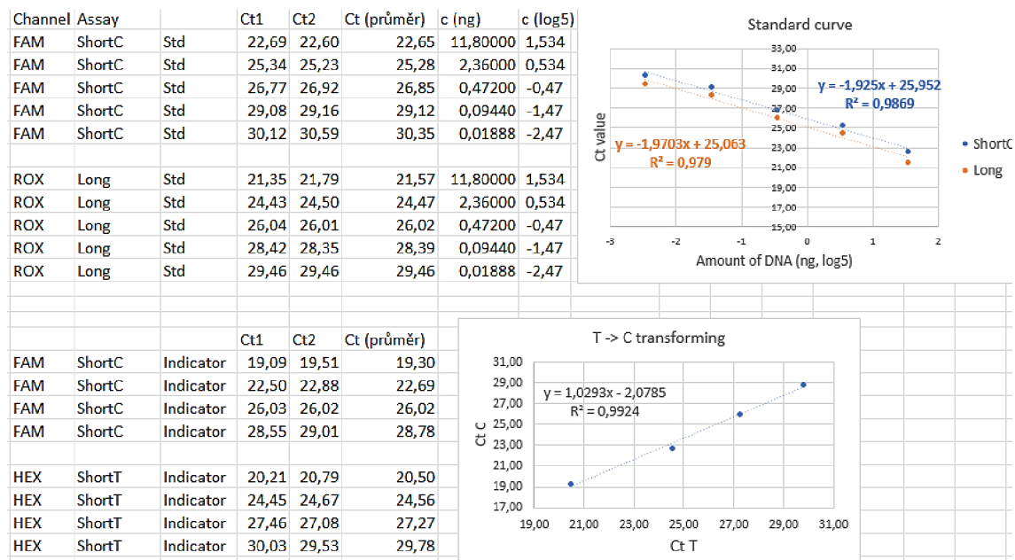
Obrázek 11 Ukázka standardů (výše) a C- T- indikátorů (níže) u experimentu pro evaluaci konverze vzorků po bisulfitové konverzi s rozdílnými amplifikačními přístupy. Standardy i indikátory byly měřeny v duplikátech (Ct1 a Ct2). Ct hodnoty u standardů i indikátorů jsou v pořádku.
