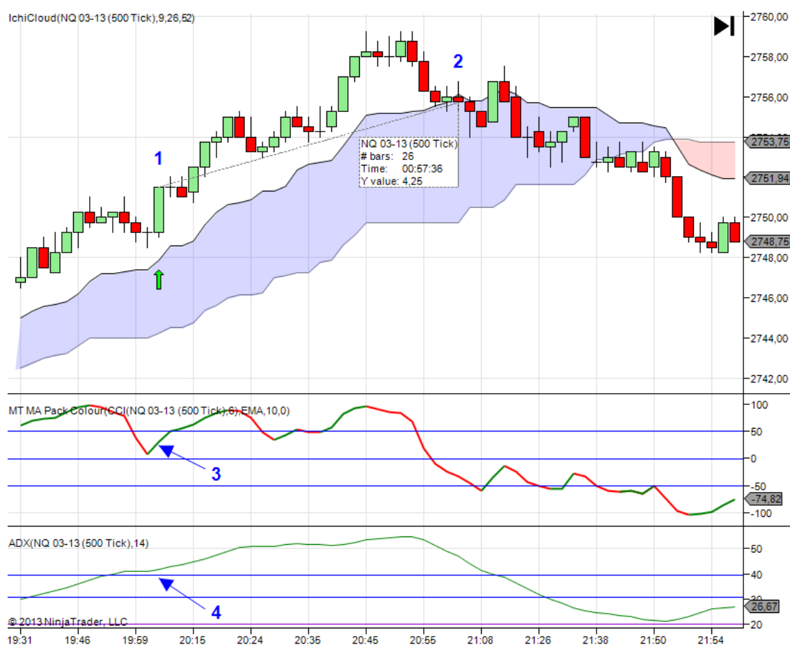
Obr. č. 15: Ukázka patternu ADX30 Long (Zdroj: vlastní)
