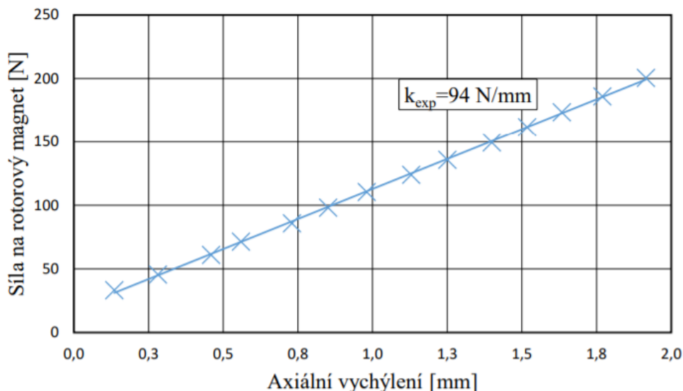
Obrázek 11: Experimentální měření závislosti působící síly na výchylce rotorového magnetu, provedené v práci [9]
