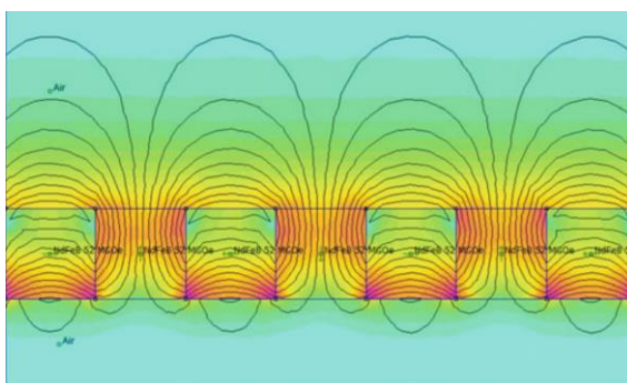
Obrázek 5: Magnetický tok magnetu s Halbachovým uspořádáním [6]
