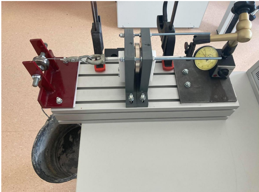
Obrázek 10: Měřicí sestava pasivního axiálního magnetického ložiska
