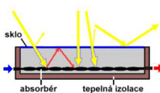
Obrázek 24 – Schéma plochého kolektoru [63]
