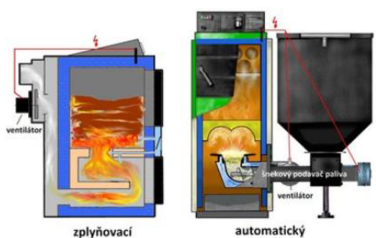
Obrázek 6 – Zplyňovací a automatický kotel na tuhá paliva [28]
