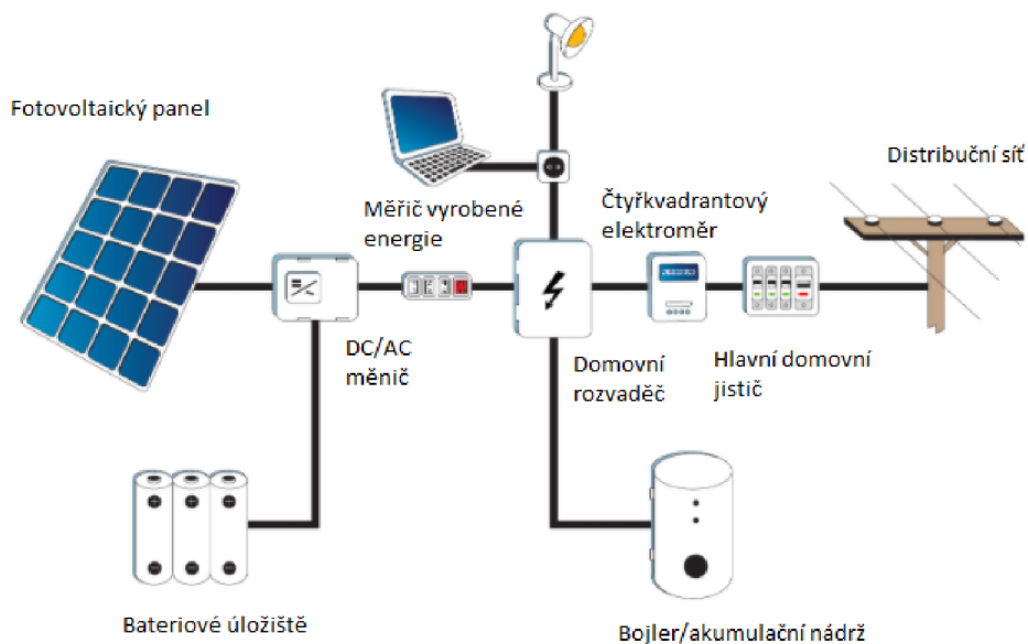
Obrázek 26 – Schéma domácího rozvodu elektřiny s fotovoltaickou elektrárnou [68]
