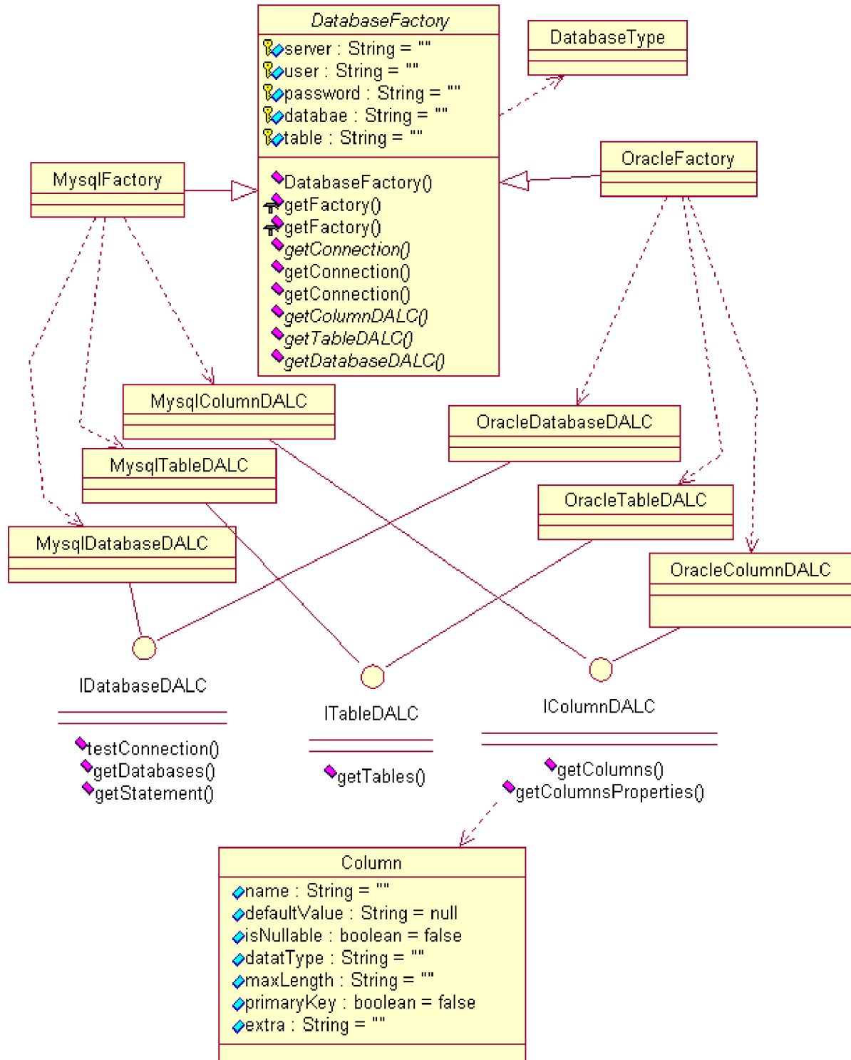
Obrázek 9: Implementovaný návrhový vzor Abstract Factory
