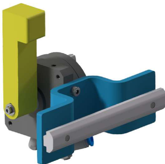
Obr. 95) Upínač palety
