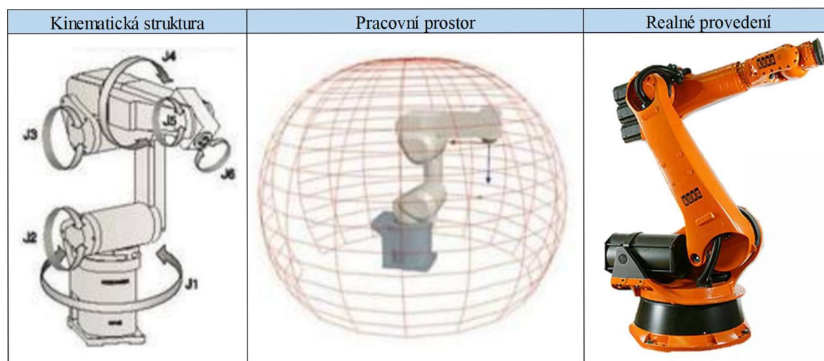
Obr. 5) Šestiosý robot [3][6]
