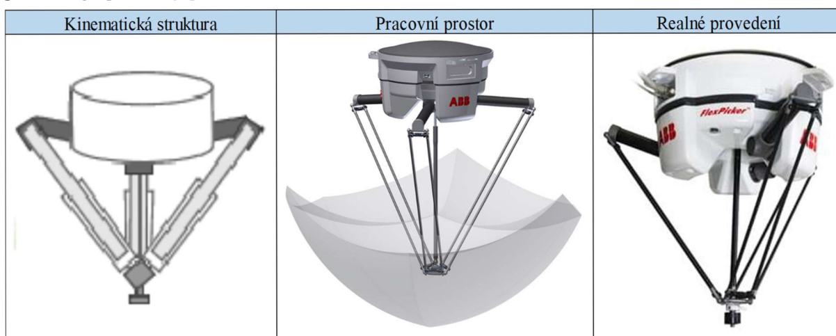
Obr. 4) Delta roboty [4][5]
