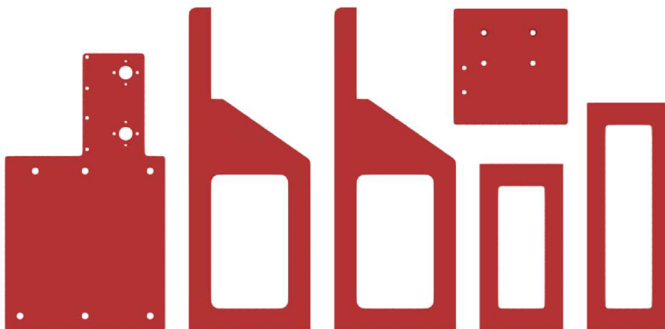
Obr. 59) Desky těla
