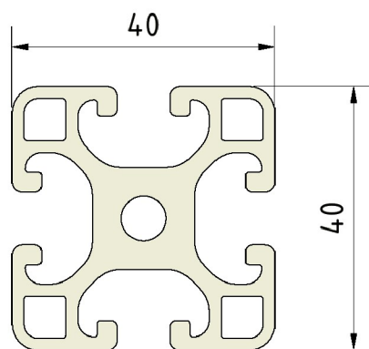
Obr. 55) Průřez profilu [36]
