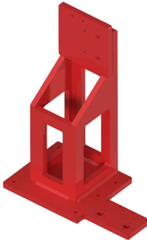
Obr. 60) Tělo manipulátoru
