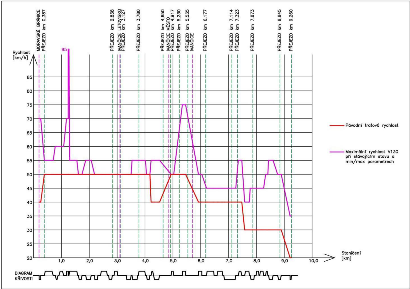
Obrázek 5 - Graf č.4 Stavající stav, minimální/maximální parametry, rychlost V130
