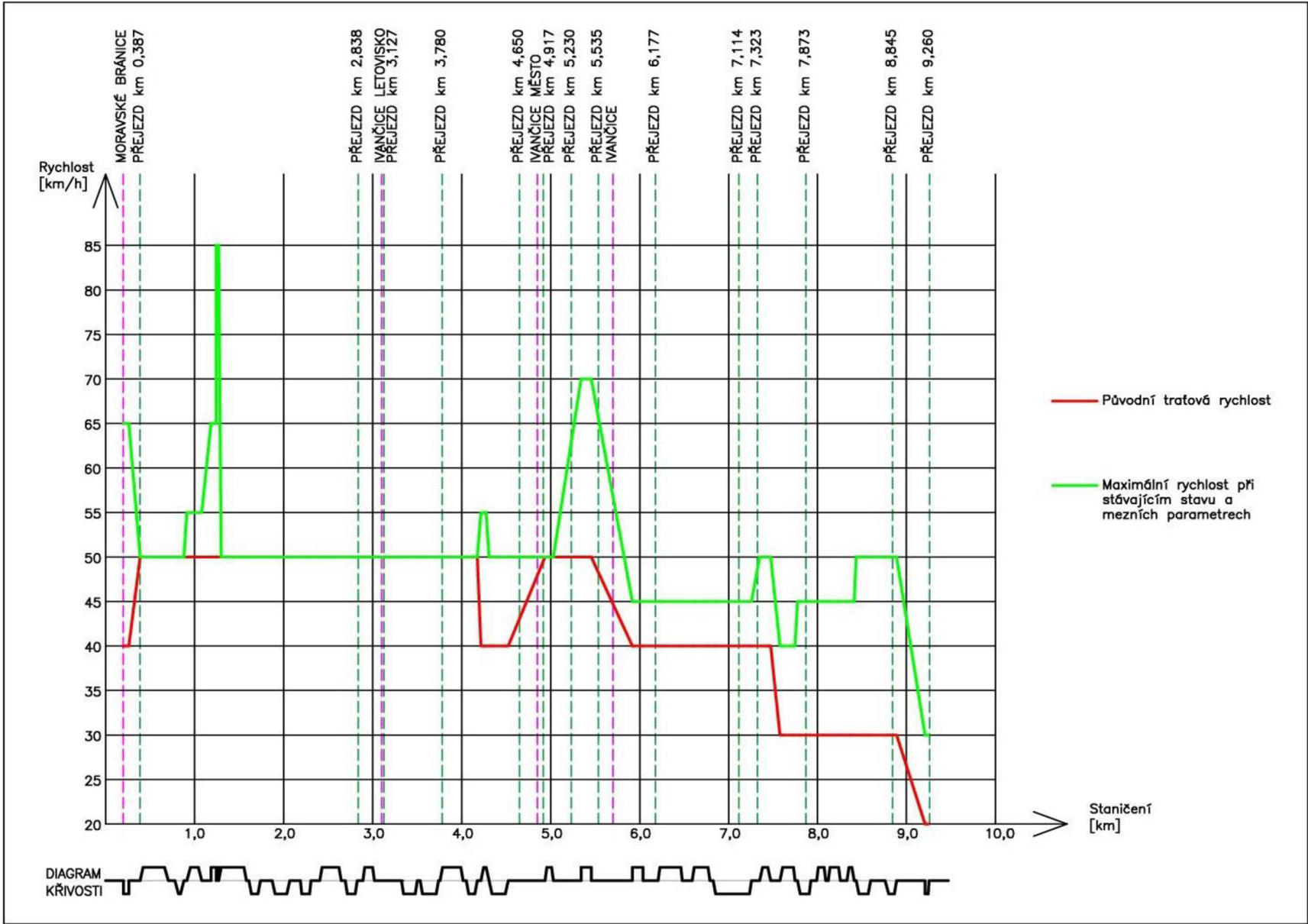
Obrázek 2 – graf č.1, stávající stav, mezní parametry, tratová rychlost
