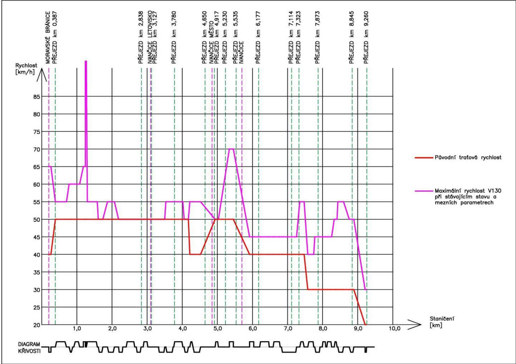
Obrázek 3 - Graf č.2. Stávající stav, mezní parametry, rychlost V130
