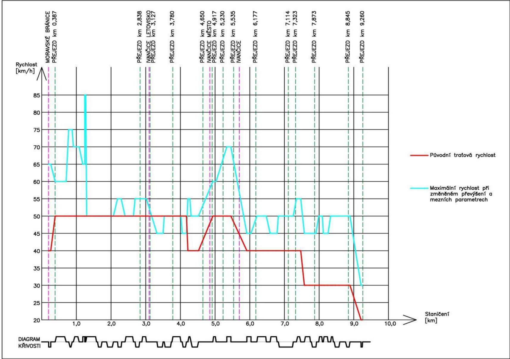
Obrázek 6 - Graf č.5 Změněné převýšení, mezní parametry, tratová rychlost
