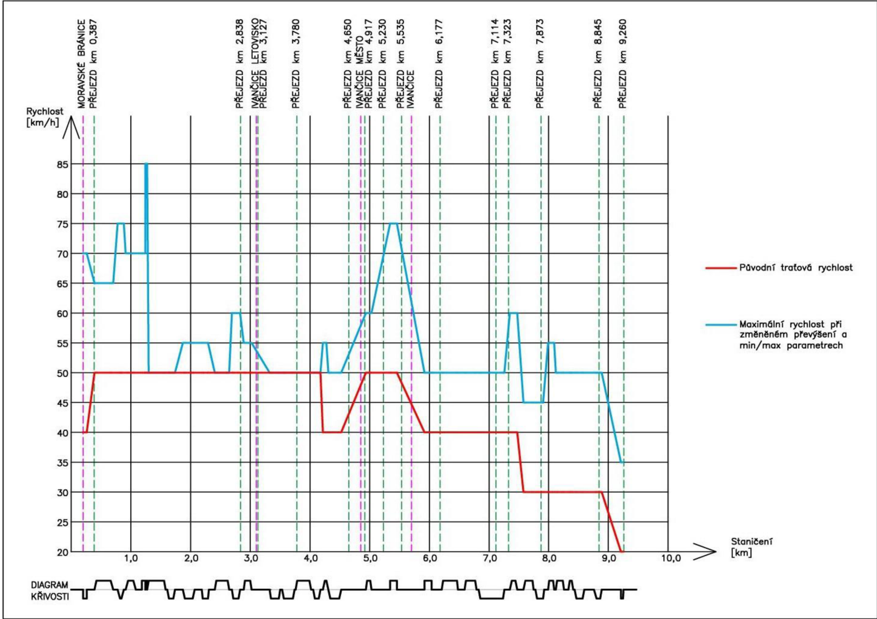
Obrázek 8 - Graf č. 7 Změněné převýšení, minimální/maximální parametry, traťová rychlost
