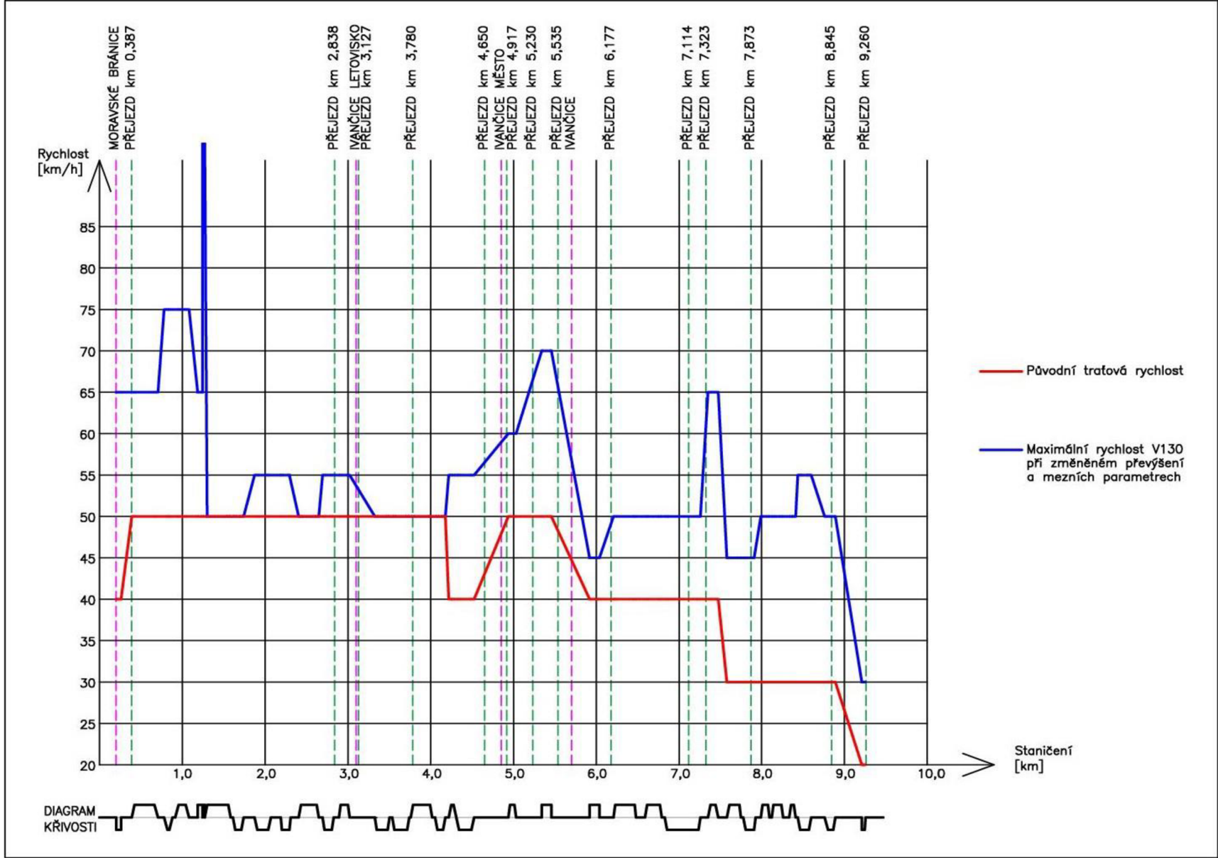
Obrázek 7 - Graf č.6 Změněné převýšení, mezní parametry, rychlost V130
