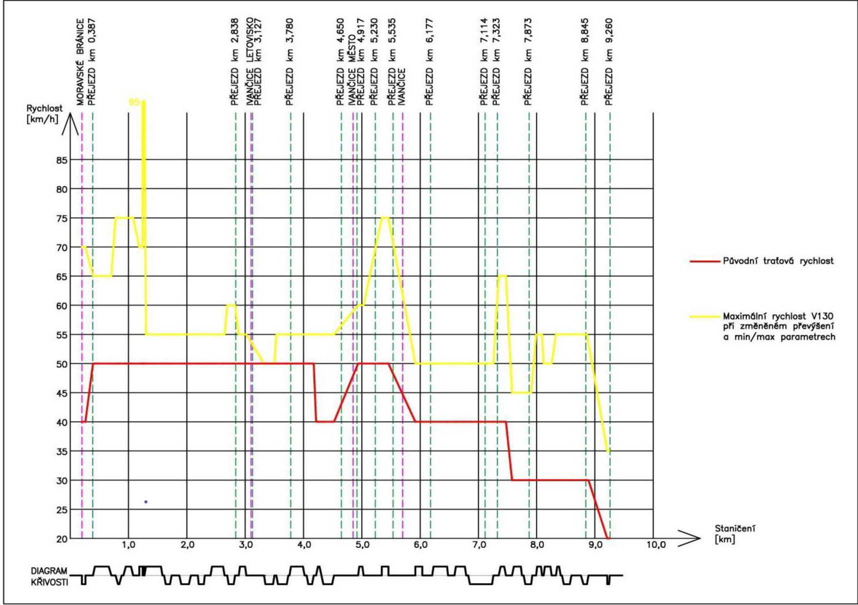
Obrázek 9 - Graf č.8 Změněné převýšení, minimální/maximální parametry, rychlost V130
