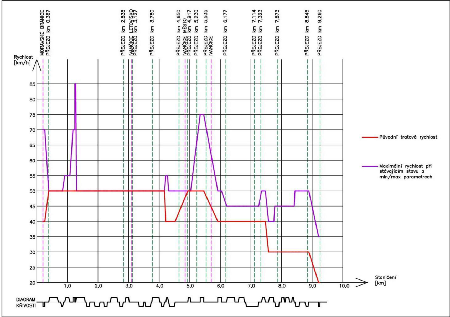
Obrázek 4 - Graf č.3 Stávající stav, minimální/maximální parametry, tratová rychlost
