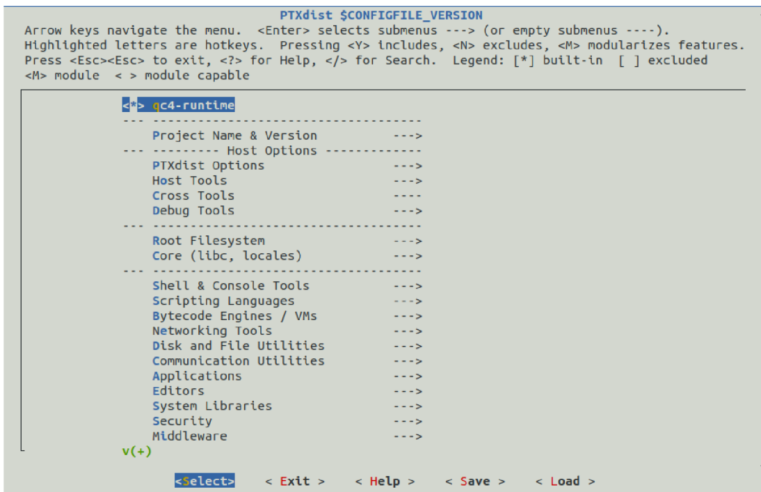
Obr. 5.8: Config Menu nástroje PTXdist
