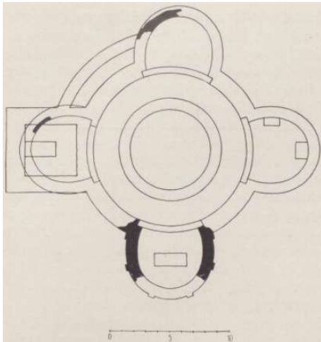
Obr. 26/ Rotunda sv. Víta, Praha, půdorys
