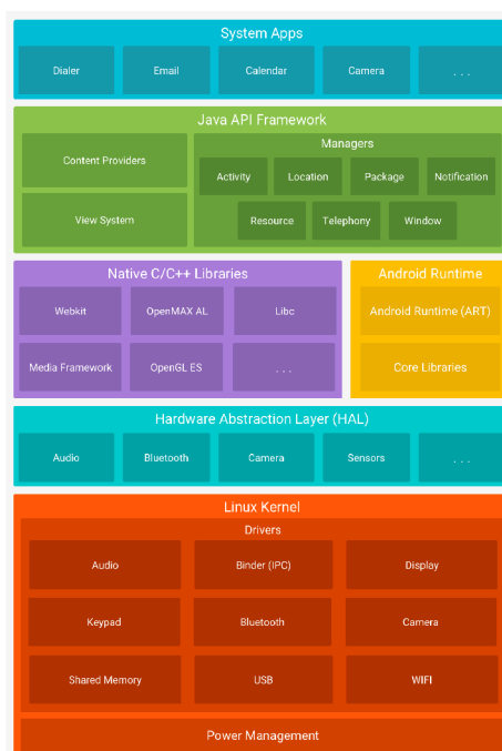
Obrázek 14: Architektura operačního systému Android
