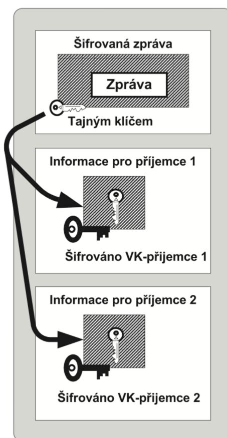
Obrázek 3: Elektronická obálka (3)
