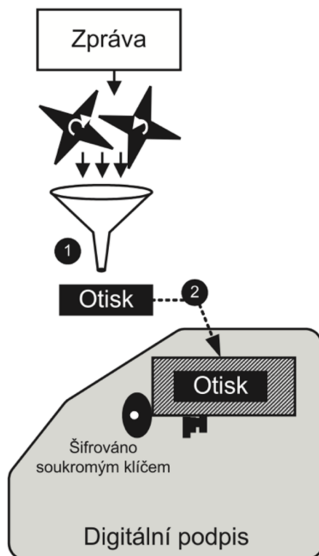
Obrázek 4: Digitální podpis (3)
