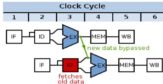
Obr. 2.2: Riešenie dátového hazardu 2
