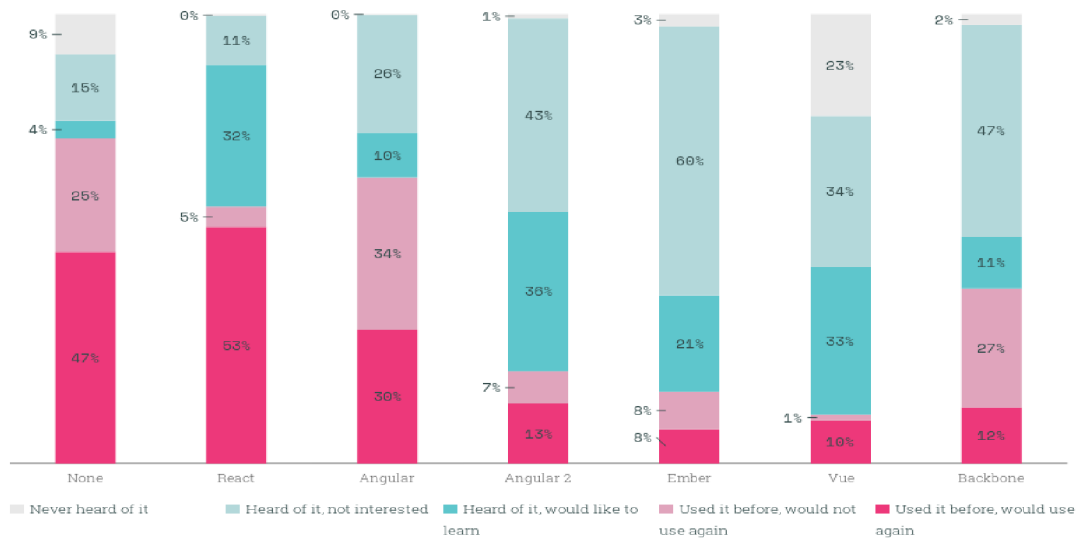
Obr. 3.1: Diagram zobrazujúci popularitu dnešných webových frameworkov 10
