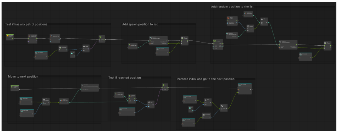
Obrázek 35 - Přehled logiky pro hlídkování Sentinela
