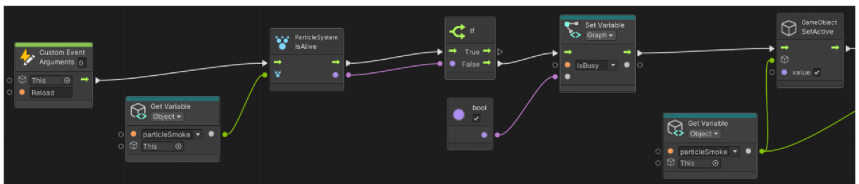
Obrázek 31 - Spuštění přebítí
