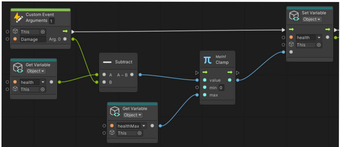
Obrázek 33 - Odečtení zdraví
