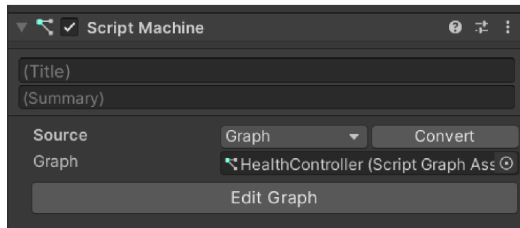
Obrázek 18 - Script Machine
