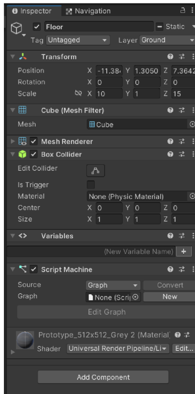
Obrázek 7 – Inspector
