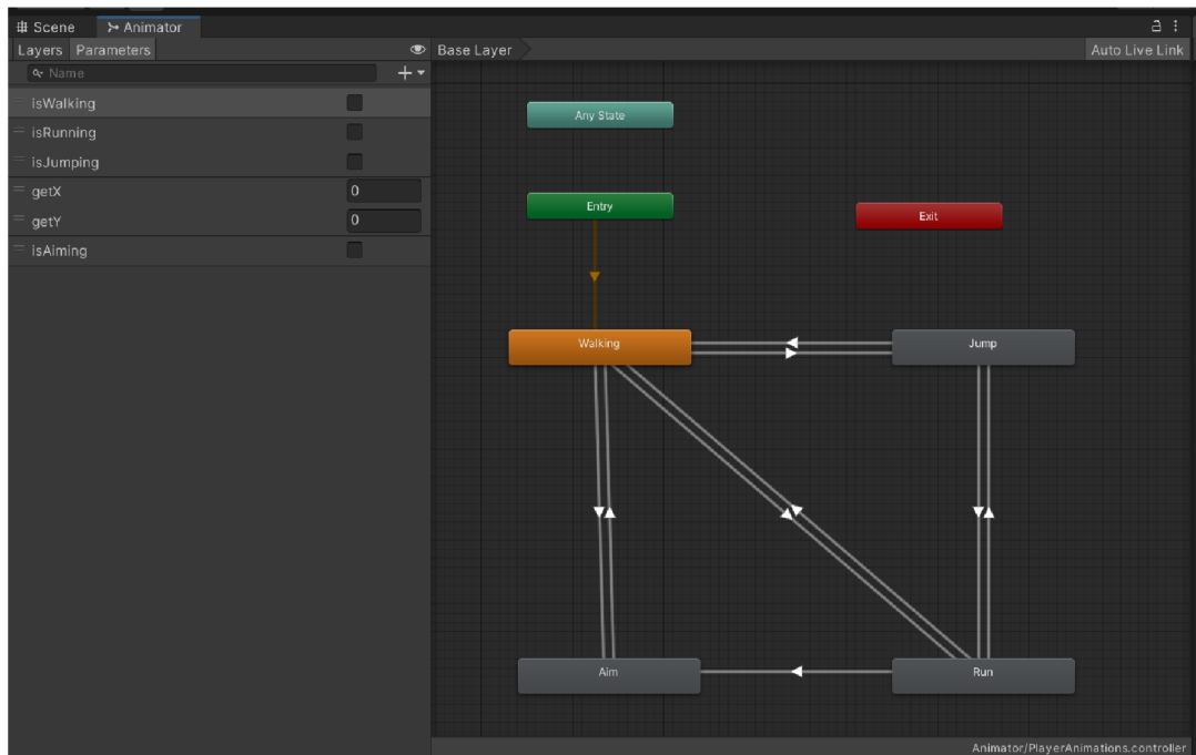
Obrázek 9 – Animator
