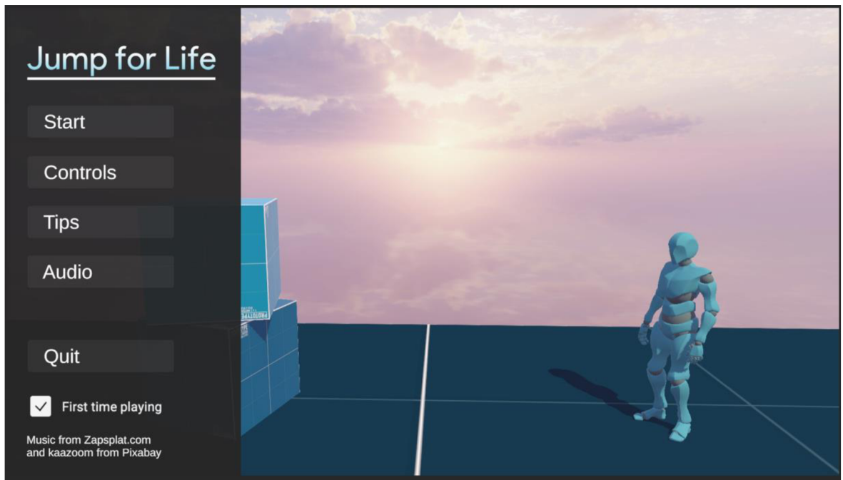
Obrázek 45 - Hlavní menu
