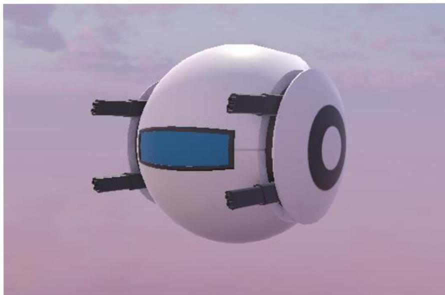
Obrázek 39 - Model Sentinel
