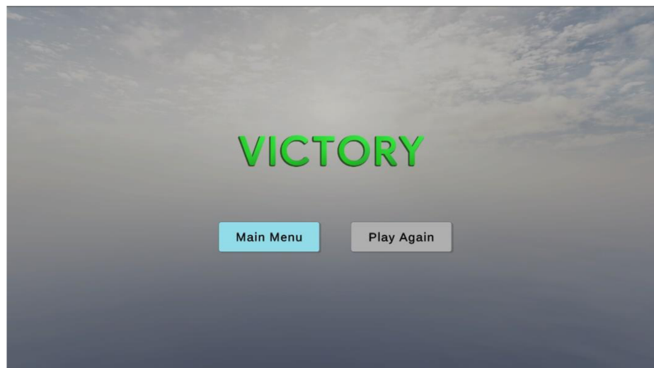
Obrázek 50 - Scéna výhry
