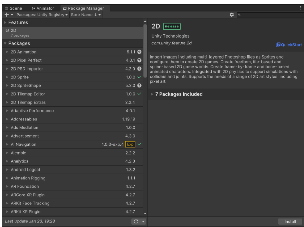
Obrázek 12 - Package Manager
