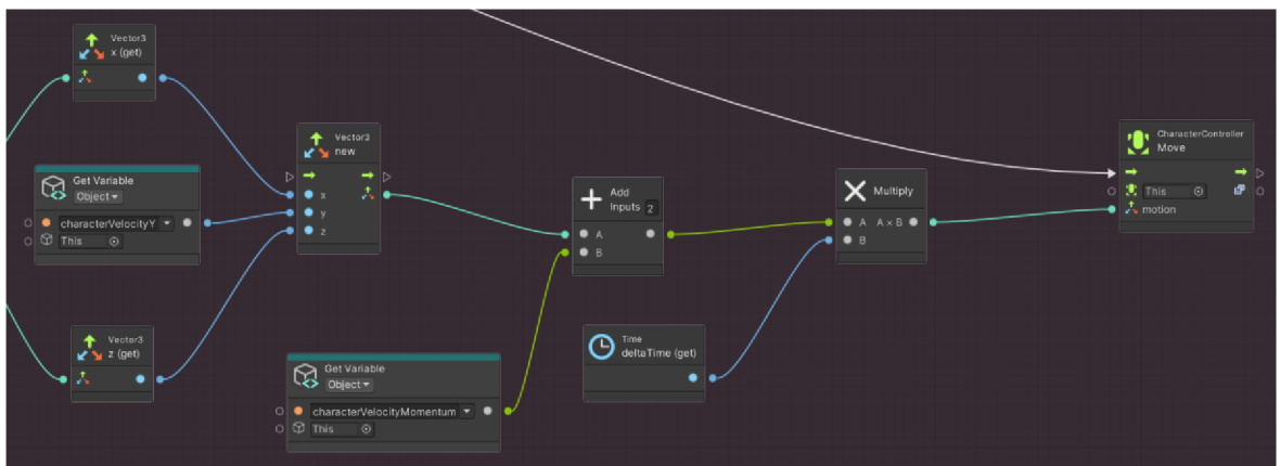
Obrázek 24 - Funkce Move
