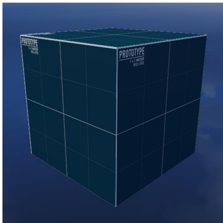
Obrázek 41 - Platforma 1x1x1
