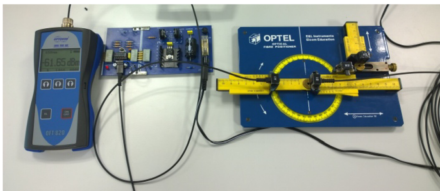
Obr. 5.1: Měření s přípravkem OPTEL
