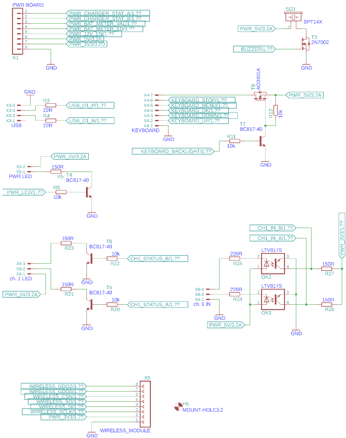
Obrázek D.11: Hlavní jednotka (druhá verze) – schéma 2/3
