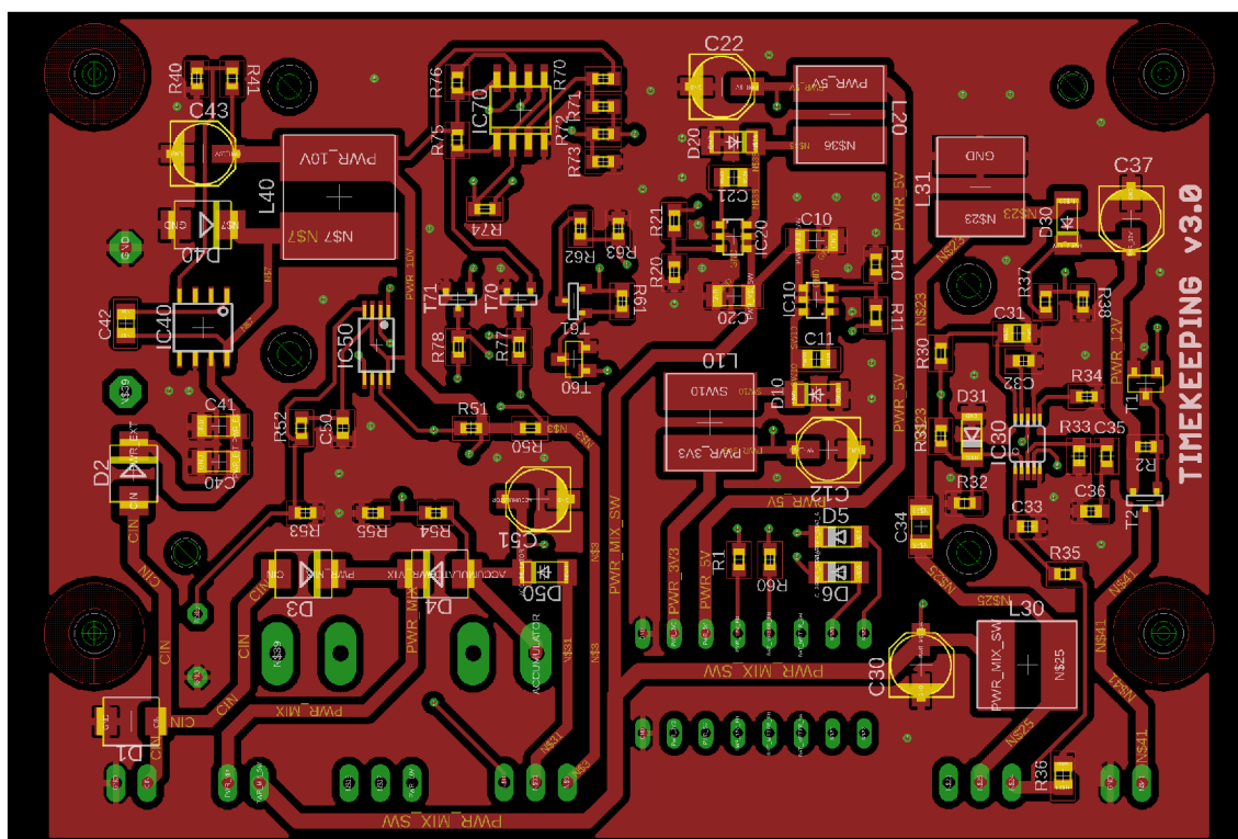
Obrázek D.9: Jednotná napájecí a nabíjecí deska (druhá verze) – DPS, měřítko 1,5:1
