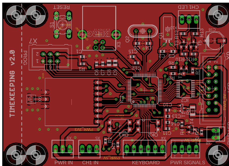
Obrázek D.2: Hlavní jednotka (první verze) – DPS, měřítko 1,5:1
