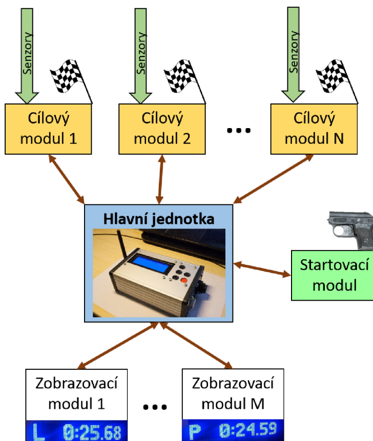
Obrázek 3.6: Navržená topologie systému časomíry
