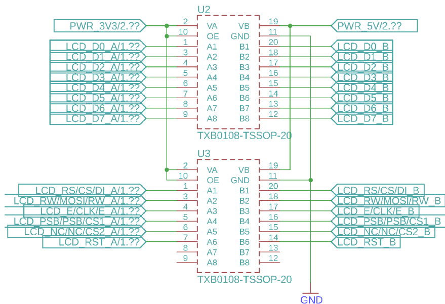
Obrázek D.12: Hlavní jednotka (druhá verze) – schéma 3/3
