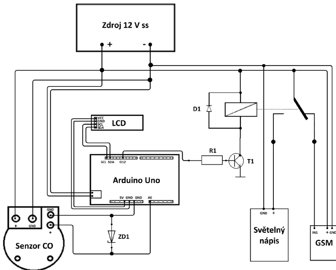
Obrázek 9 Schéma zapojení celého zařízení
