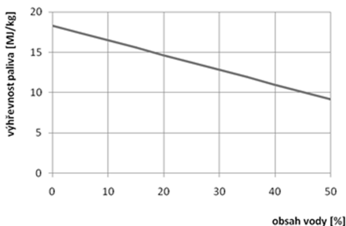
Obr. 2 Závislost výhřevnosti paliva na obsahu vody[5]
