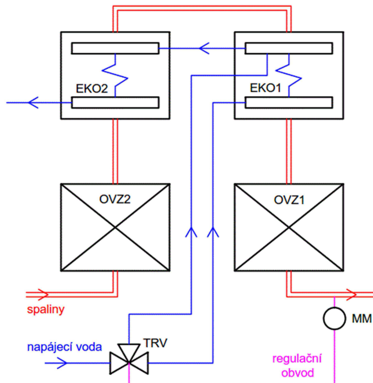
Obr. 18 Schéma regulace teploty spalin na výstupu z kotle
