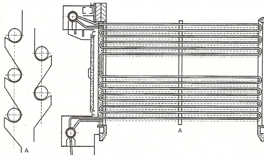
Obr. 7 Ohřívák vody [1]
