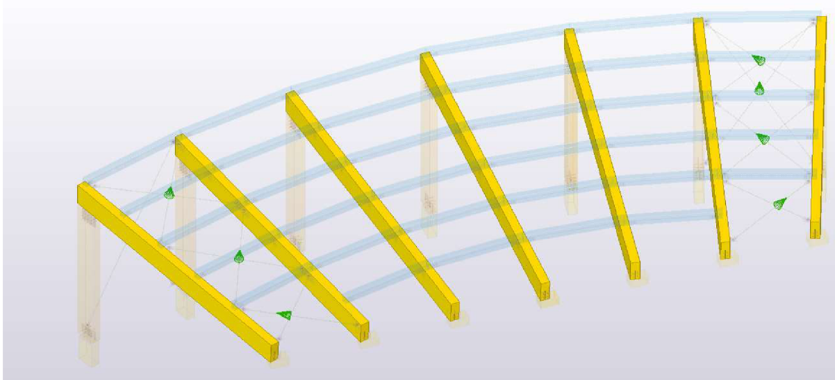
Obrázek 6 - vazníky
