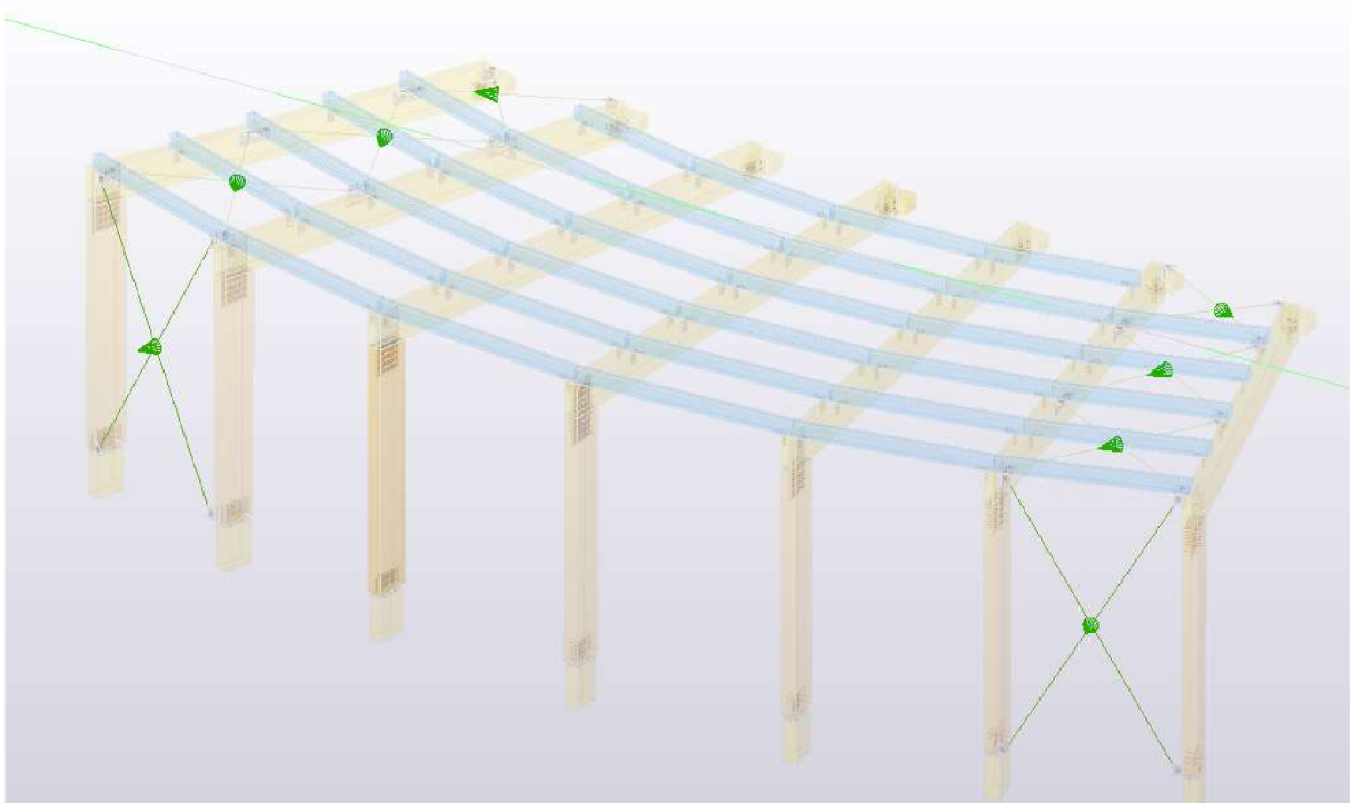
Obrázek 10 - stěnová ztužidla
