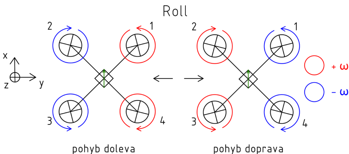
Obr. 10 – Rotace kolem osy x
