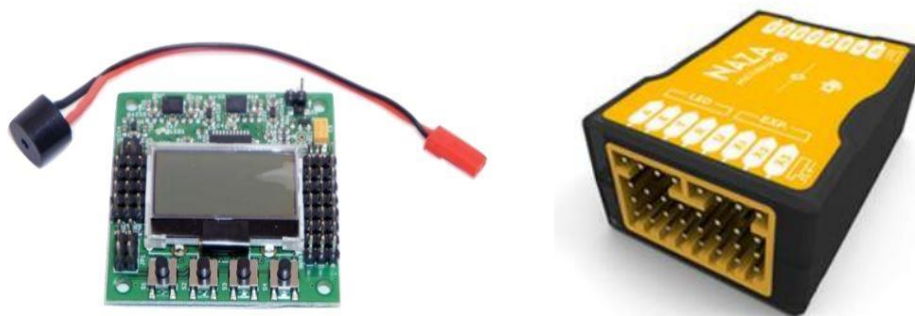
Obr. 16 – Řídící deska NAZA [23]
