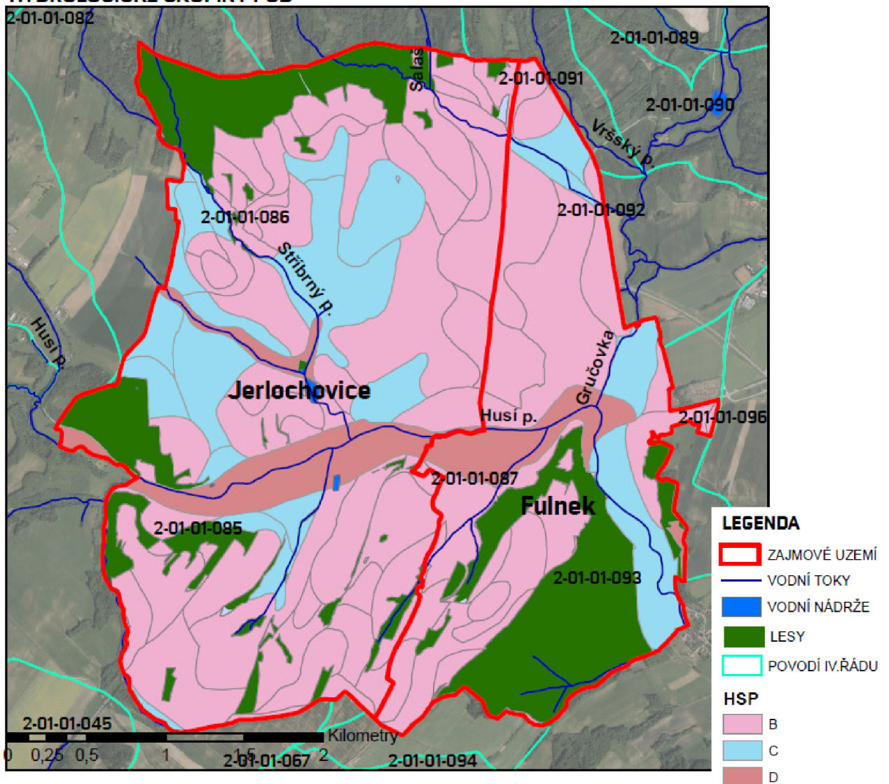
Obrázek 18 - Mapa HSP
