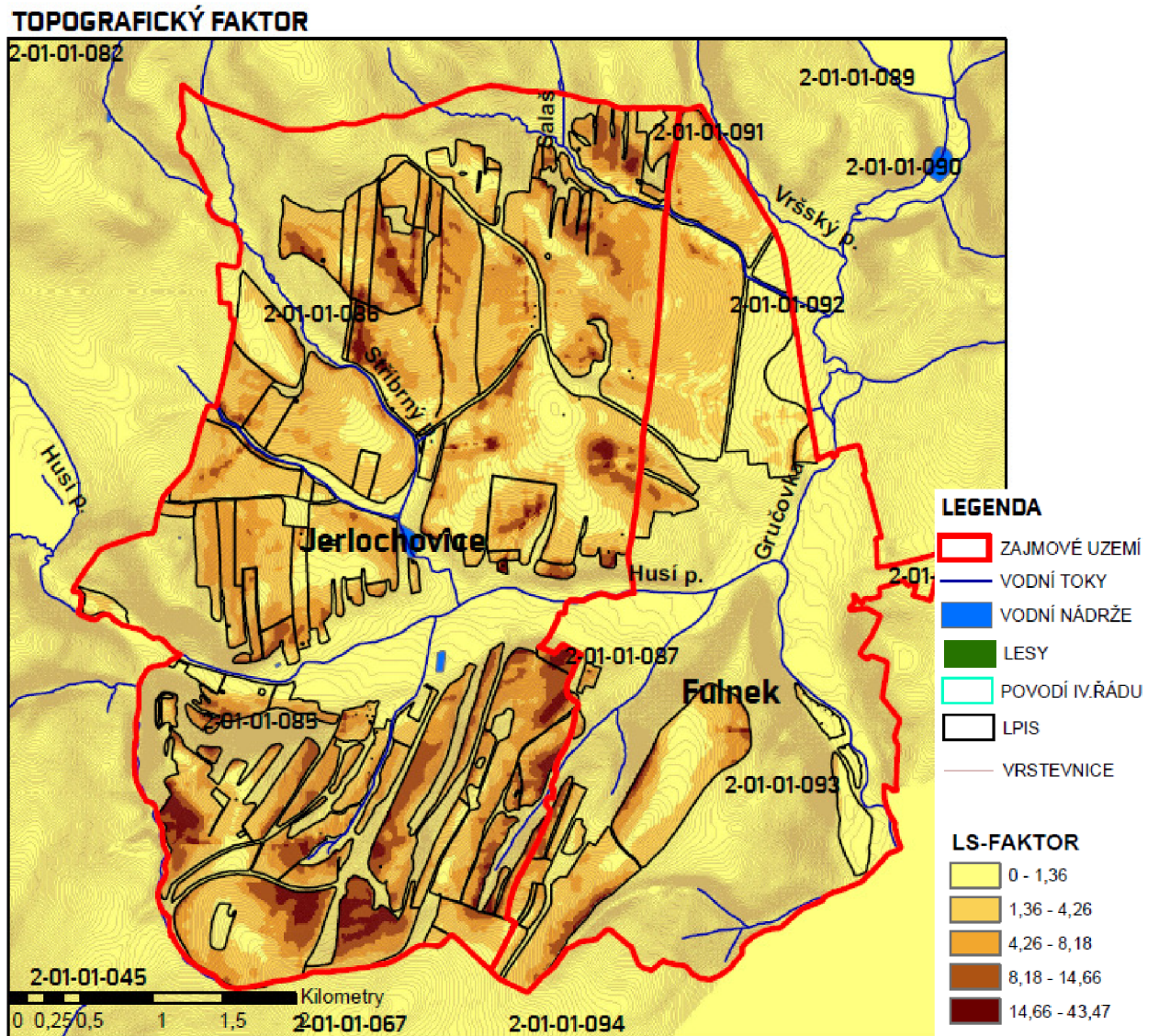
Obrázek 19 - Mapa LS-faktoru
