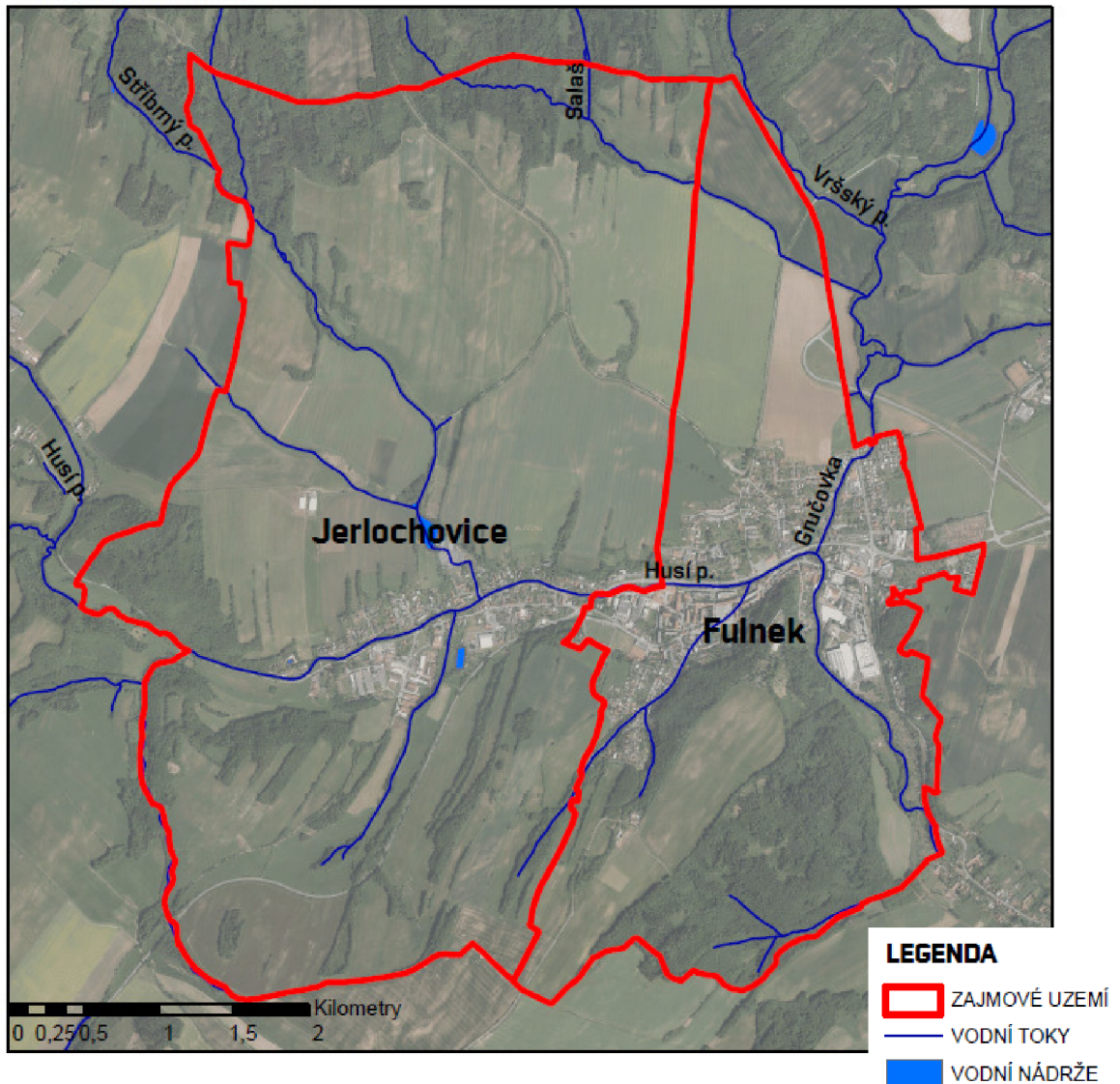
Obrázek 15 - Hydrologické poměry
