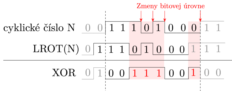
Obr. 2.7: Príklad počítania zmien bitových úrovní.
