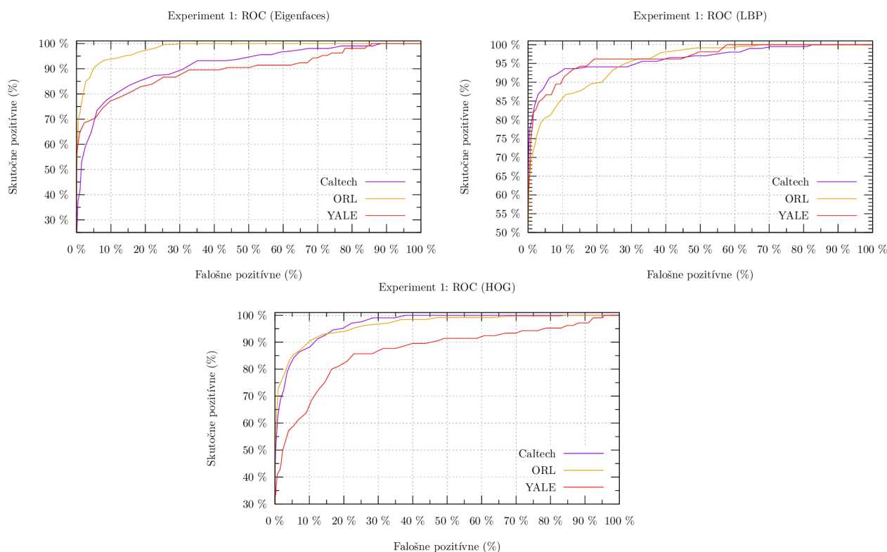
Obr. 4.4: Porovnanie ROC kriviek jednotlivých implementovaných metód pri verifikácii na troch rôznych dátových sadách.
