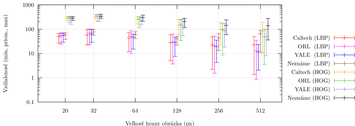
Obr. 4.11: Závislosť vzdialenosti medzi rozpoznávanou snímkou a šablónou z databázy na použitom rozlíšení snímky pri metódach LBP a HOG.
