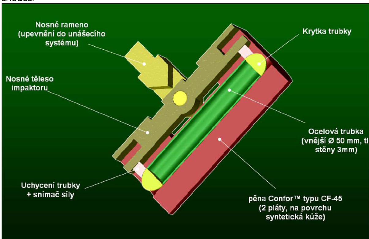
Obr. 4 Impaktor stehna [6]
