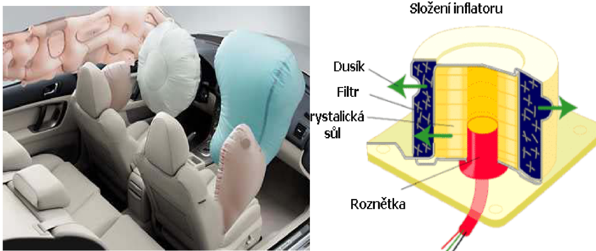
Obr. 17 Sestava airbagů a vyvíječ plynu airbagu [15]
