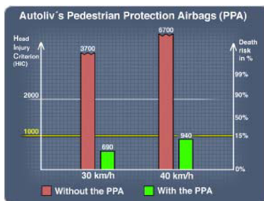
Obr. 13 Použití airbagů k ochraně chodců a jejich vliv na HIC [10]
