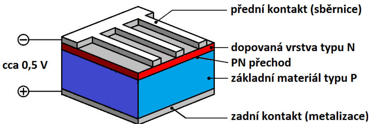
Obr. 5.1 Solární článek [29]
