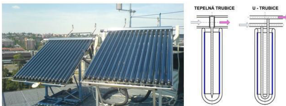
Obr. 5.4 Trubicový kolektor [34]
