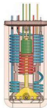
Obr. 5.6 Akumulační nádoba [34]
