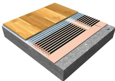
Obr. 7.4 Podlahová topná folie [45]
