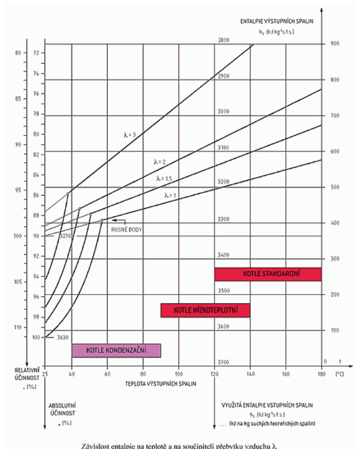
Obr. 4.2 Entalpický diagram [36]
