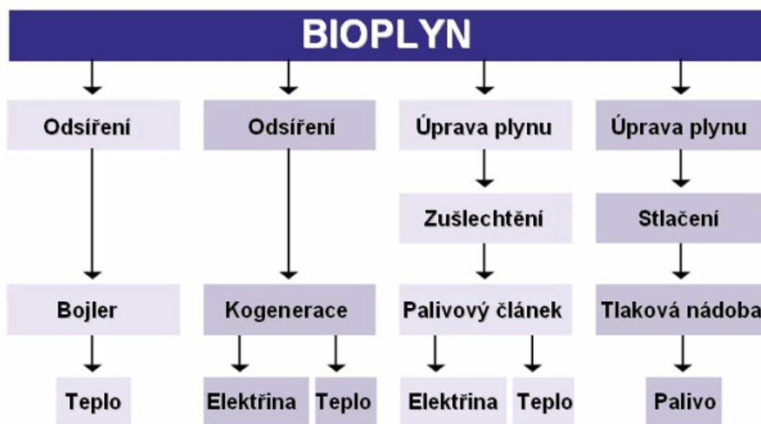
Obr. 3.6 Využití bioplynu [10]
