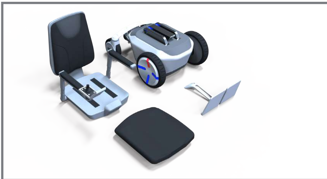
Obr. 6-59 Ukázka rozložení vozíku na dílčí komponenty
