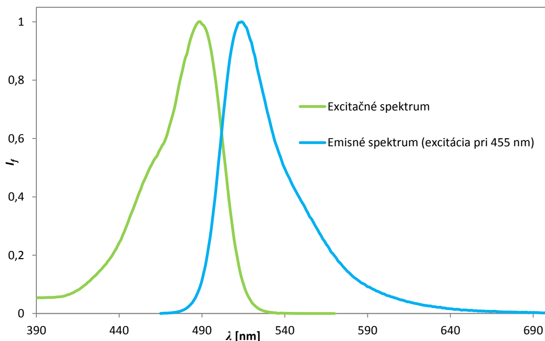
Obrázok 12: Normalizované excitačné a emisné spektra OG488 v 0,15 M NaCl s koncentráciou 8 \cdot 10^{-6} M
