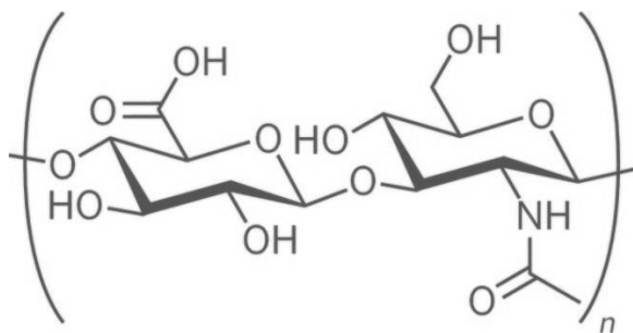
Obrázok 11: Štruktúra kyseliny hyaluronovej
