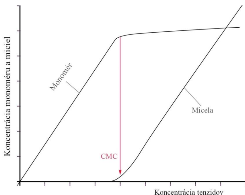
Graf 1: Zmena koncentrácie monoméru a miciel ako funkcia koncentrácií PAL. CMC - kritická micelárna koncentrácia [21]
