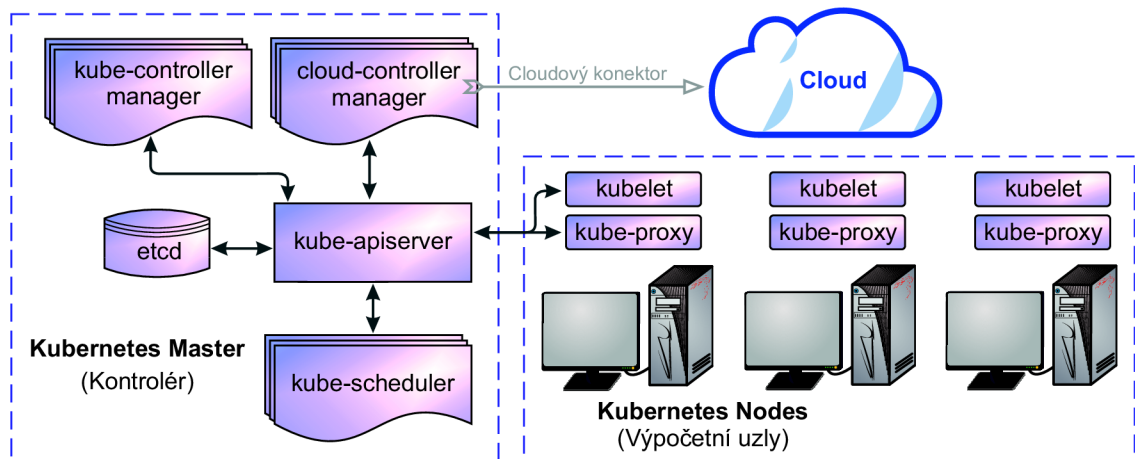
Obr. 1.6: Architektura platformy Kubernetes
