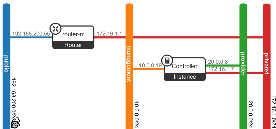
Obr. 2.1: Předpřípravená topologie
