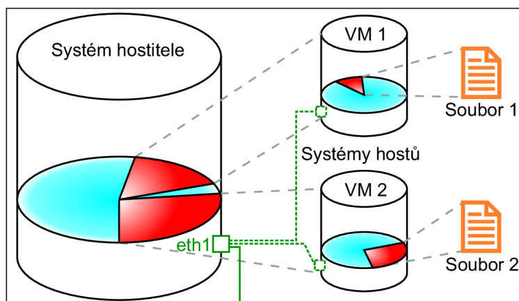
Obr. 1.1: Virtualizace systému
