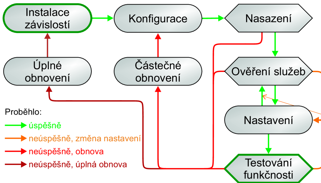
Obr. 2.3: Stavový diagram instalace a zprovoznění OpenStacku pomocí nástroje kolla-ansible
