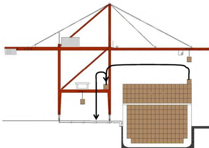
Obr. 26 Jeřáb s jednou kočkou, dvojitým zdvihem a pevnou překládací plošinou [13]
