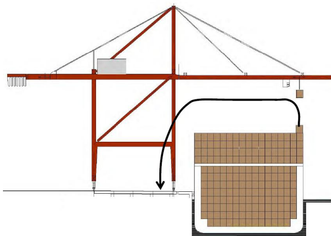
Obr. 25 Jeřáb s jednou kočkou a jedním zdvihem [13]
