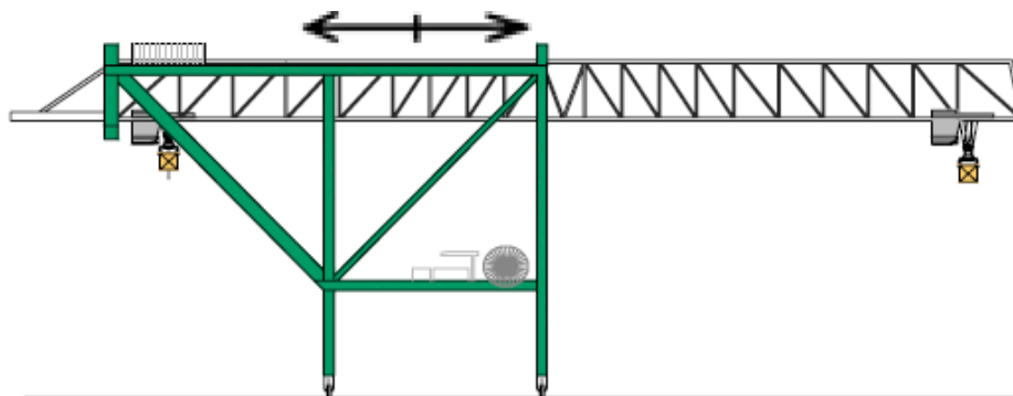
Obr. 21 Nízkoprofilový jeřáb [23]
